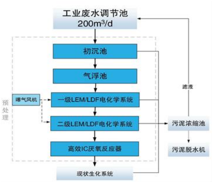
图 7.1.2-1 废水处理工艺流程图
