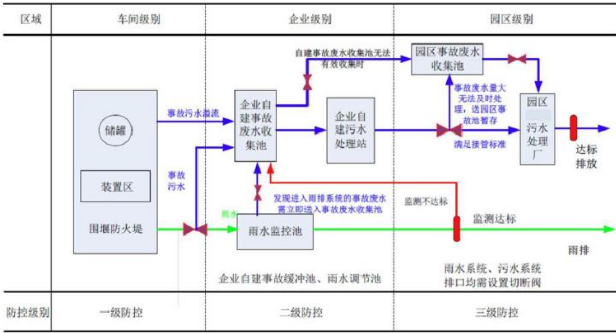
图 6.9.4-1 项目厂区事故状态下切断措施
