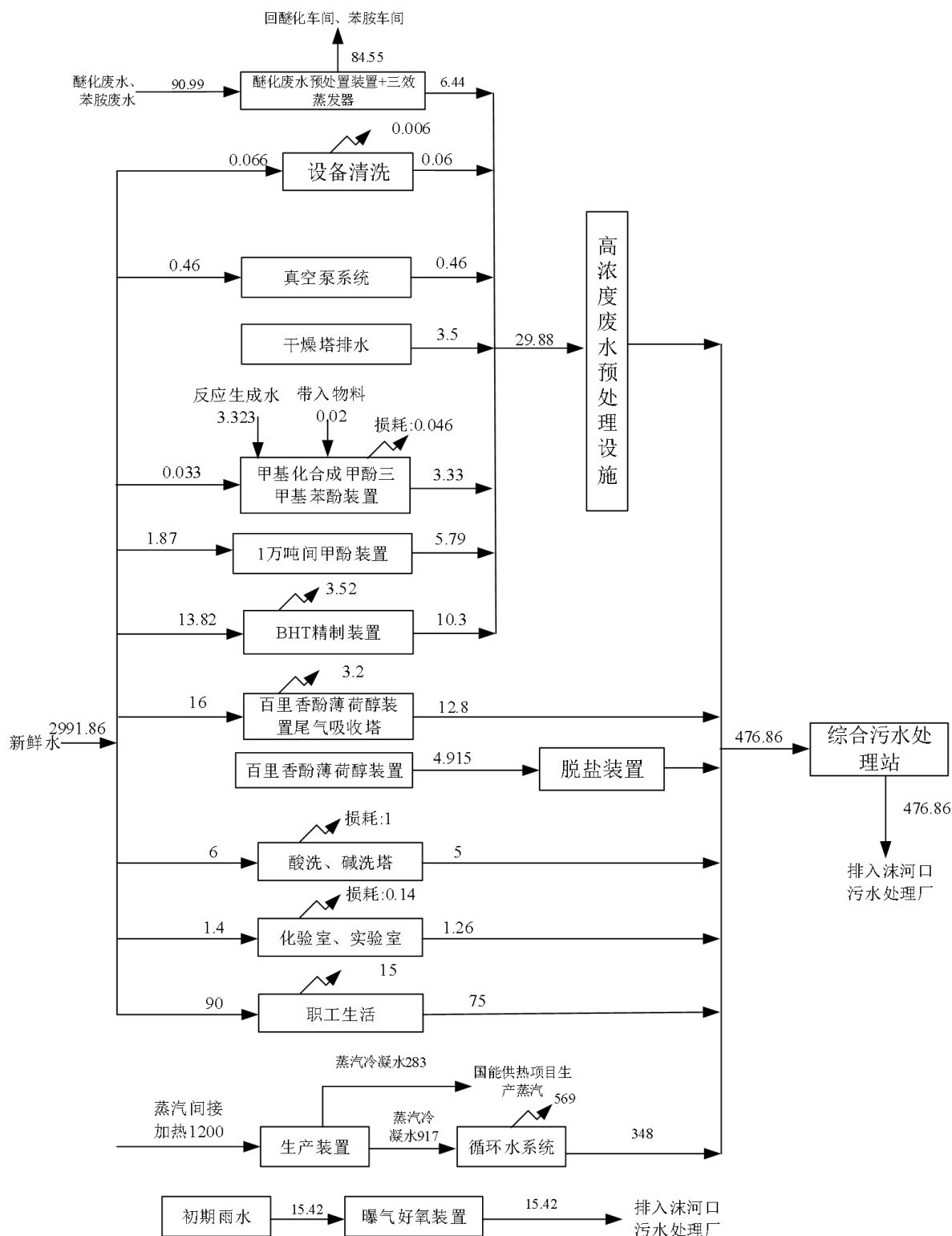
图 2.1.4-1 海华科技现有工程水平衡图 单位: m³/d
