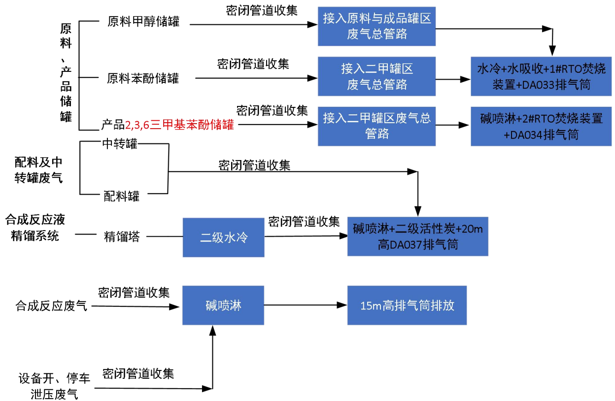
图 7.2-1 废气收集方案示意图
