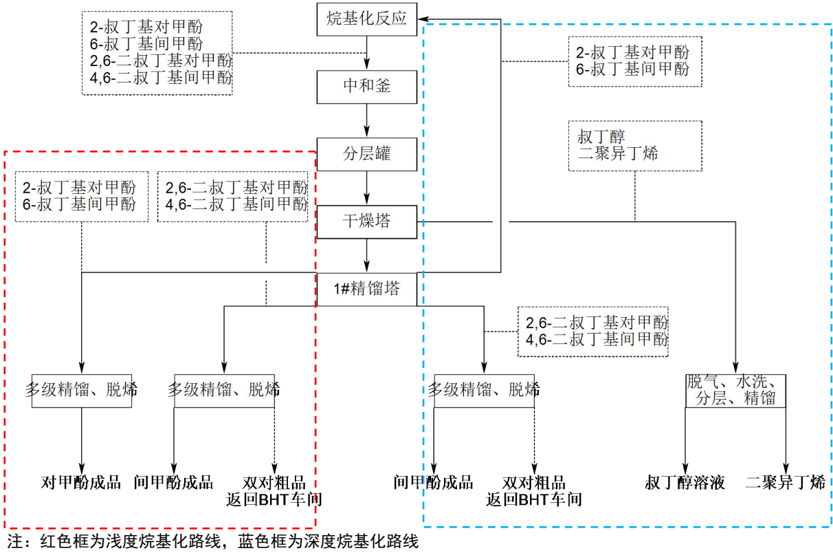
图 2.2-1 间甲酚车间技改前后工艺路线示意图
