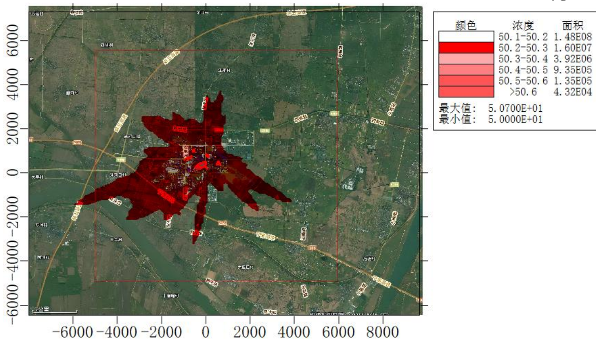
图 5.2.3-7 叠加现状浓度、拟建、在建污染源后甲醇日平均贡献浓度分布图 单位: \mu\text{g}/\text{m}^3
