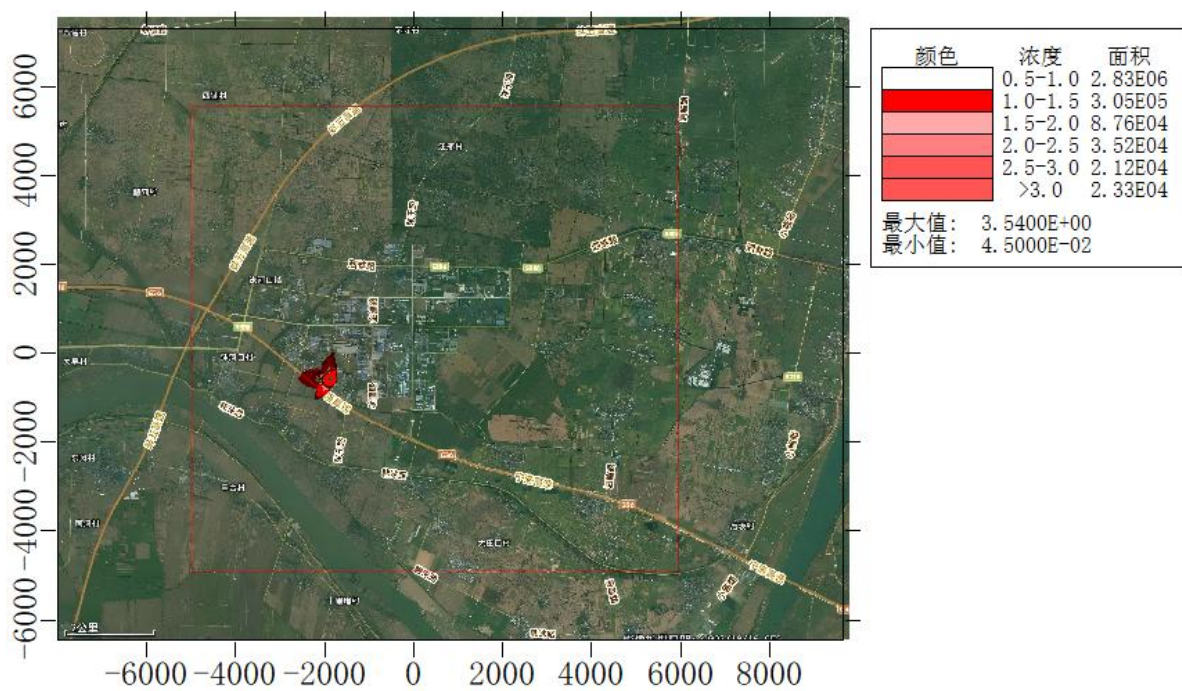
图 5.2.3-8 叠加现状浓度、拟建、在建污染源后酚类小时平均贡献浓度分布图 单位: \mu\text{g}/\text{m}^3
