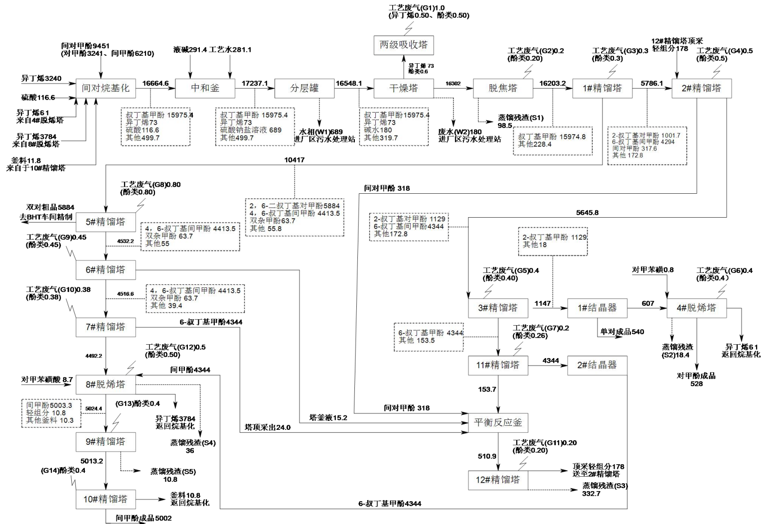
图 2.2-2 间甲酚车间浅度烷基化工艺物料平衡图
