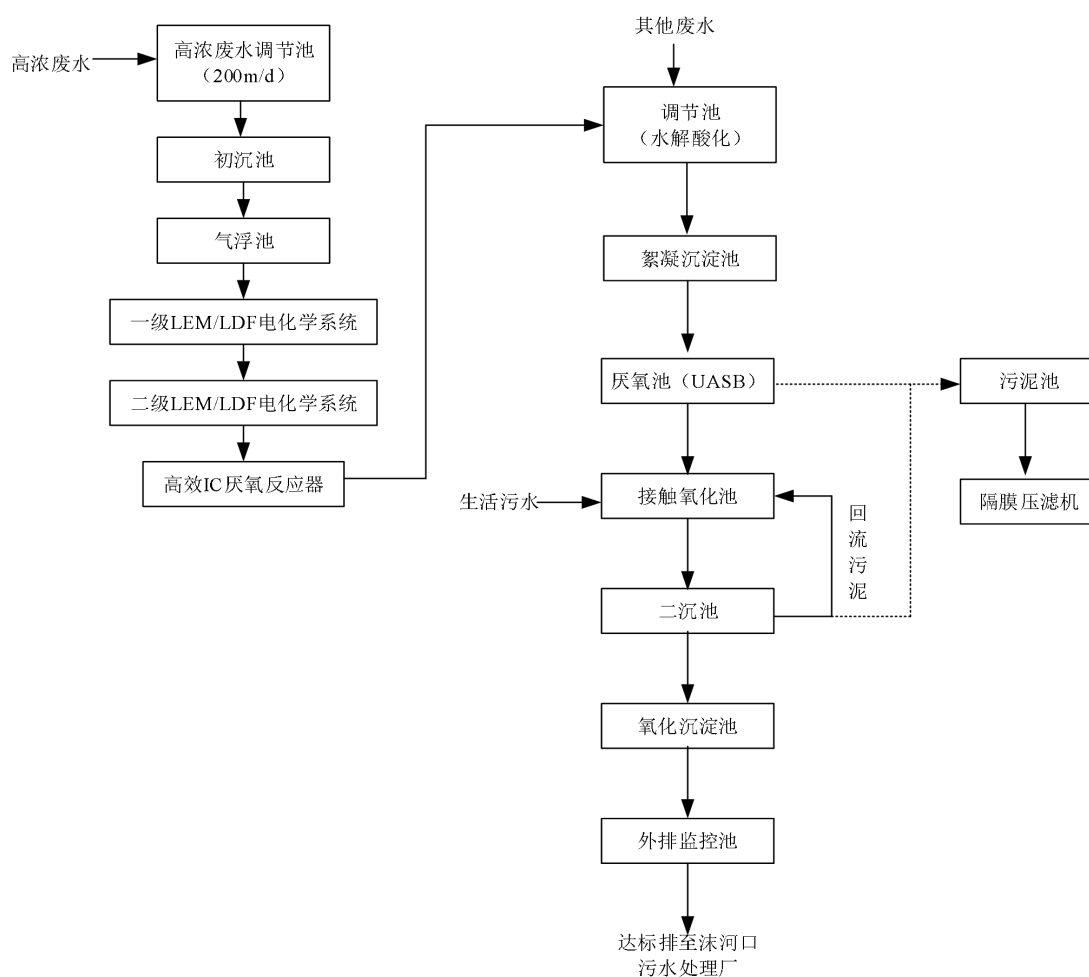
图 2.1.4.2 海华科技污水处理工艺流程图
