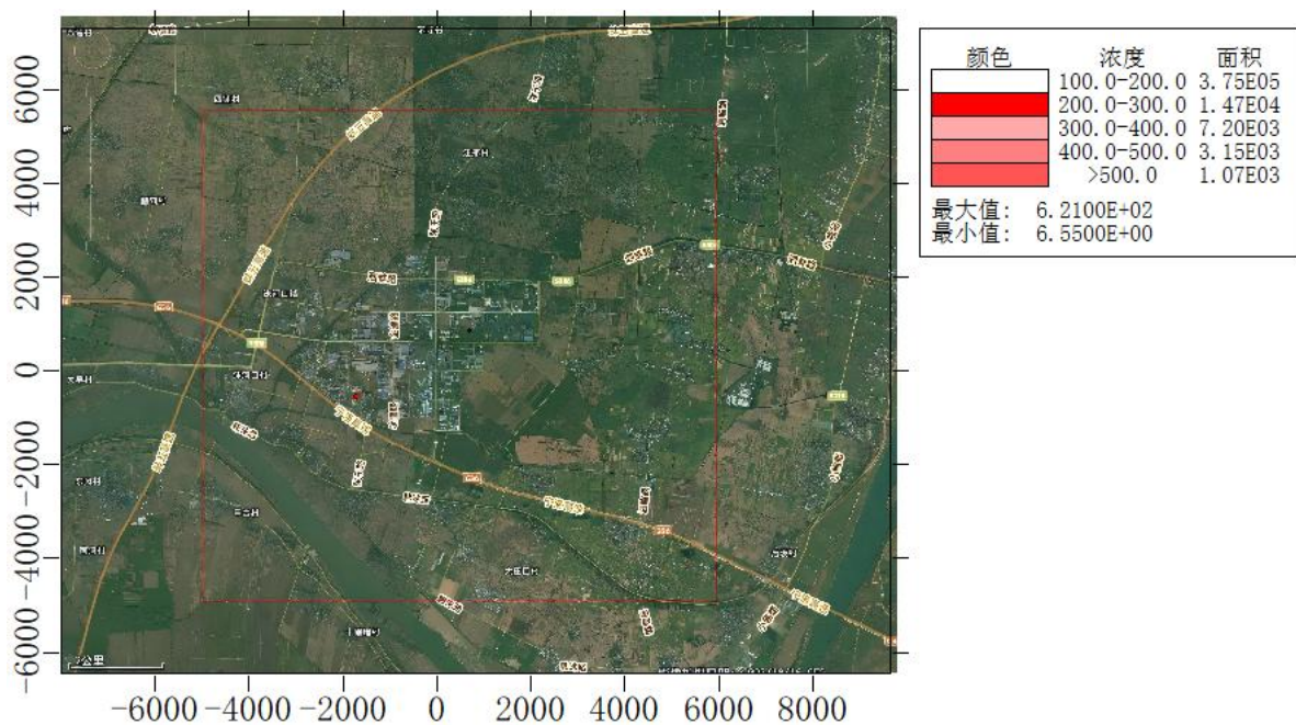
图 5.2.3-5 叠加现状浓度、拟建、在建污染源后非甲烷总烃小时平均贡献浓度分布图 单位: \mu\text{g}/\text{m}^3
