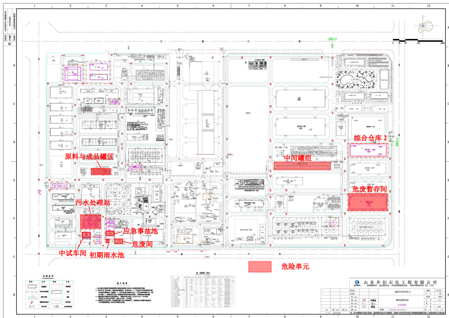
图 6.6.4-1 危险单元分布图
