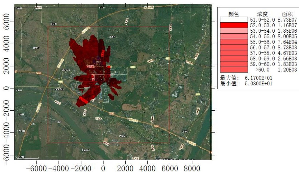
图 5.2.3-6 叠加现状浓度、拟建、在建污染源后甲醇小时平均贡献浓度分布图 单位: \mu\text{g}/\text{m}^3
