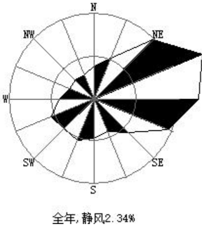
图 5.2.1-1 蚌埠市风向玫瑰图（静风频率 2.34%）
