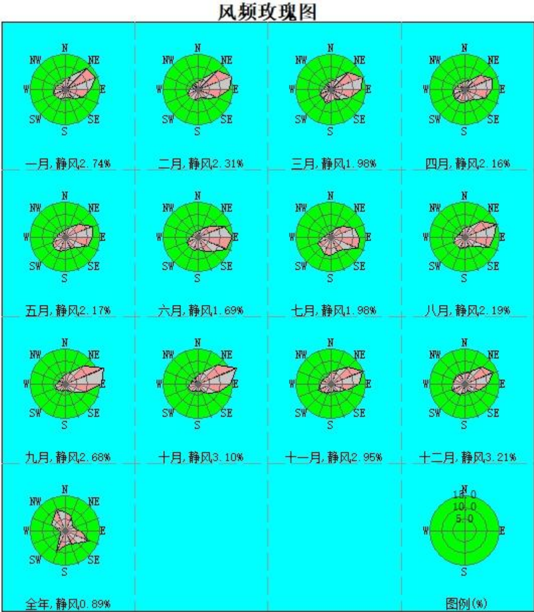
图 5.2.1-4 2023 年蚌埠市气象站风向频率玫瑰图
