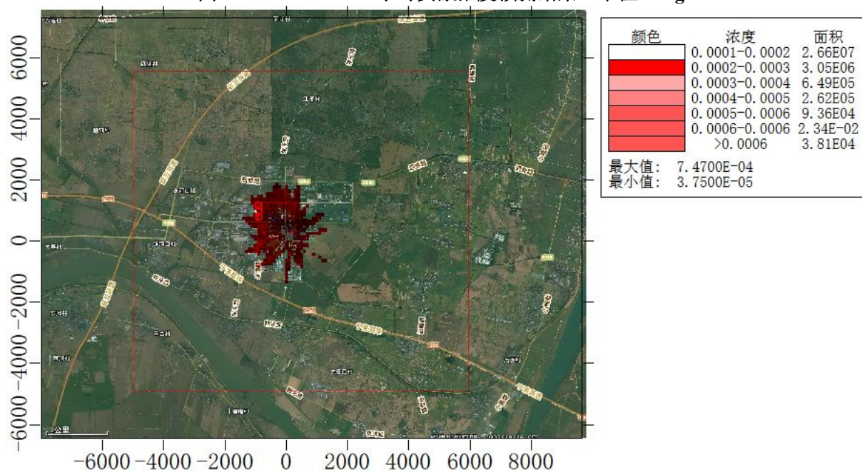
图 5.2.3-2 甲醇小时贡献浓度预测结果 单位: \text{mg}/\text{m}^3
