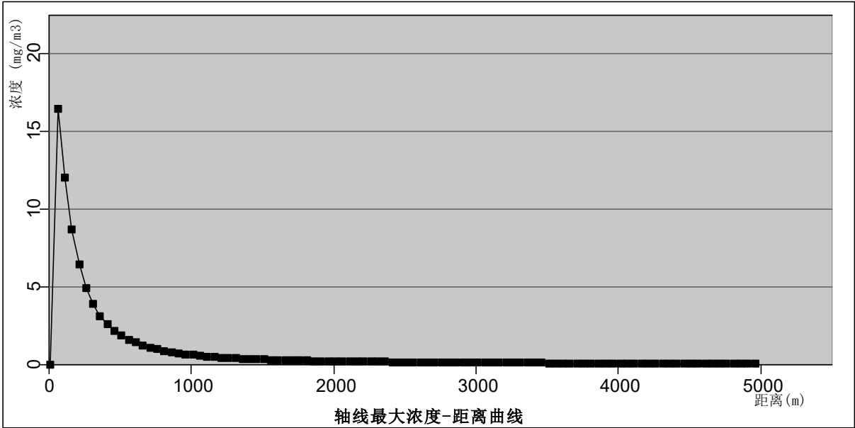
图 6.8.1-2 最不利气象条件下事故状况下风向甲醇不同距离最大浓度
