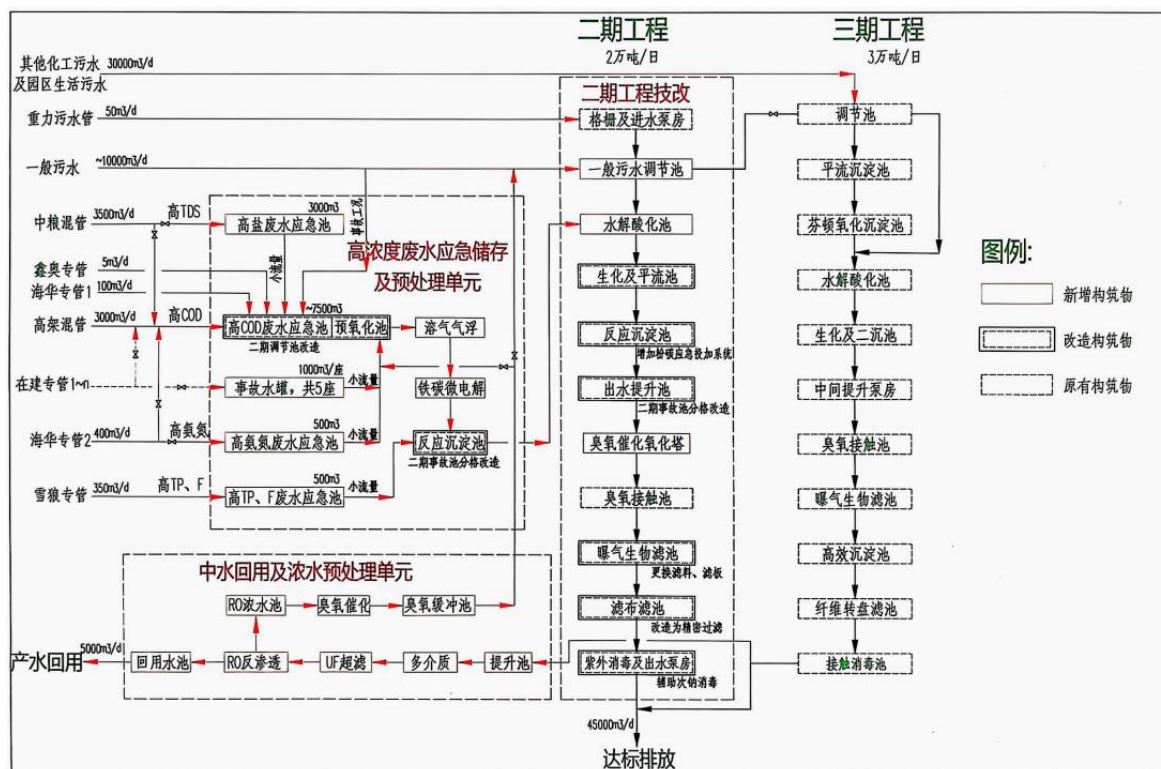
图 7.1.3-3 沫河口污水处理厂改造后工艺流程示意图
