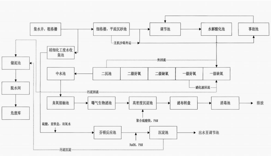
图 7.1.3-2 现状洙河口污水处理厂三期工程工艺流程图
