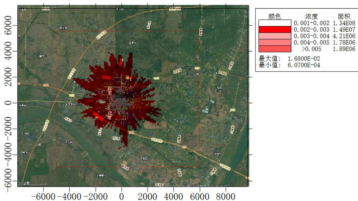
图 5.2.3-1 NMHC 小时贡献浓度预测结果 单位: \text{mg}/\text{m}^3
