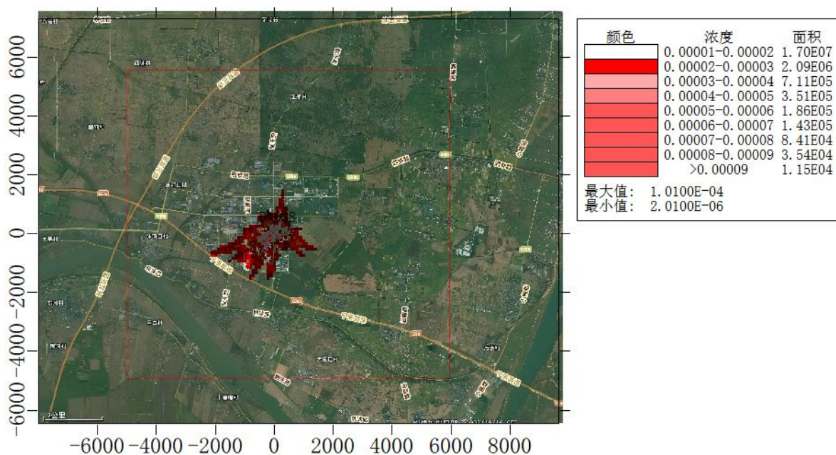
图 5.2.3-3 甲醇日均贡献浓度预测结果 单位: \text{mg}/\text{m}^3
