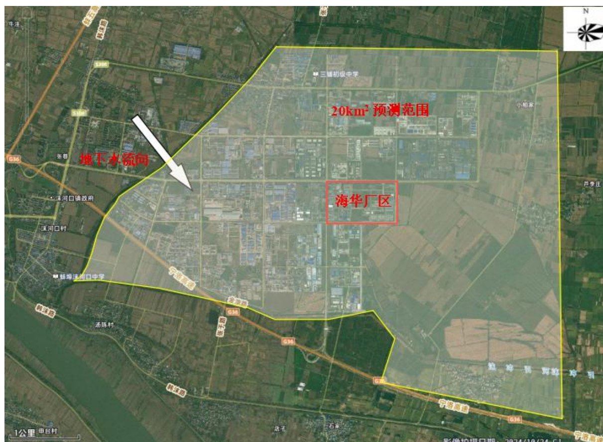
图 5.5.2-2 地下水预测范围图
