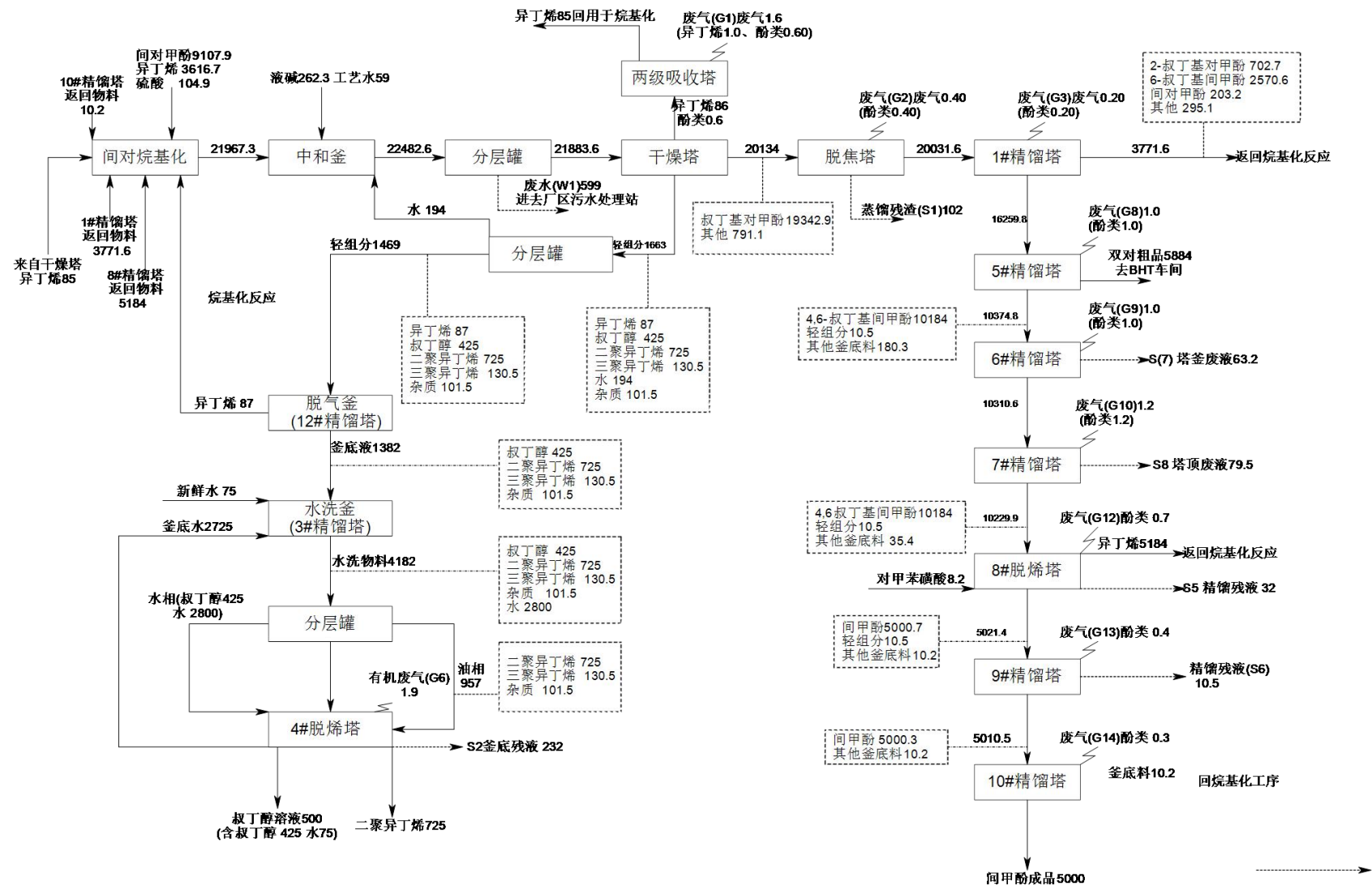
图 2.2-3 间甲酚车间生产（深度烷基化）生产工艺流程、产排污节点及物料平衡图 t/a
