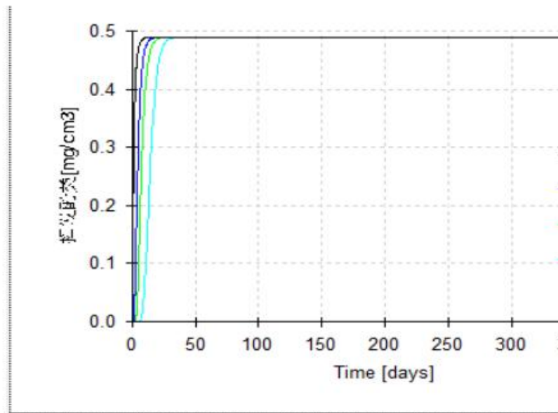
图 5.6.4-1 渗透时间与挥发酚浓度关系图
