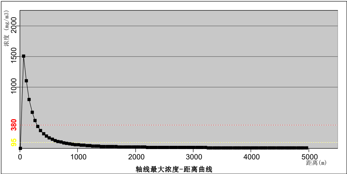
图 6.8.1-3 最不利气象条件下事故状况下风向间 CO 不同距离最大浓度
