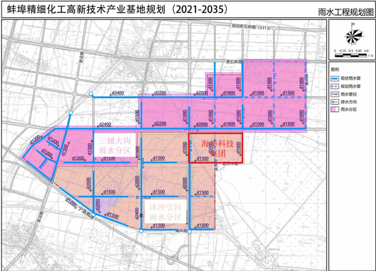
图 6.3.2-1 园区雨水排放示意图
