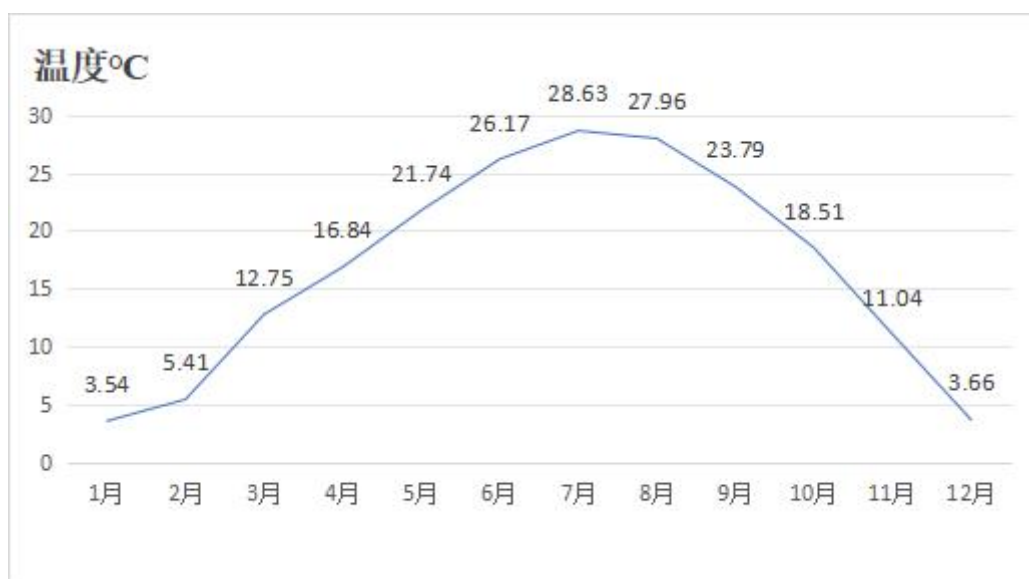
图 5.2.1-2 2023 年蚌埠市气象站年平均温度月变化
