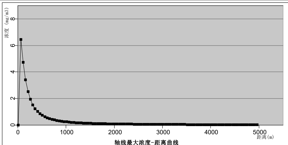
图 6.8.1-1 最不利气象条件下事故状况下风向苯酚不同距离最大浓度
