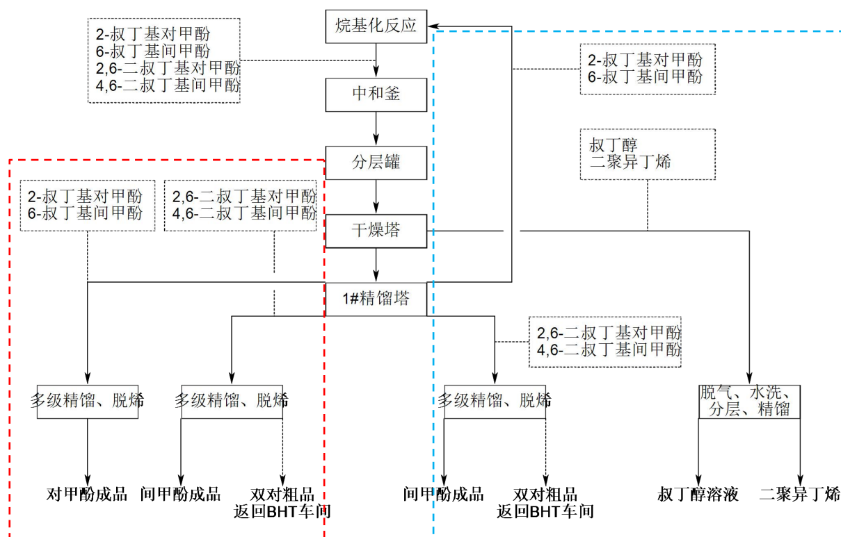
图 2.2-1 间甲酚车间技改前后工艺路线示意图
