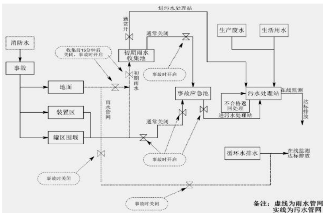
图 6.2.3-1 现有项目事故废水收集调储系统示意图
