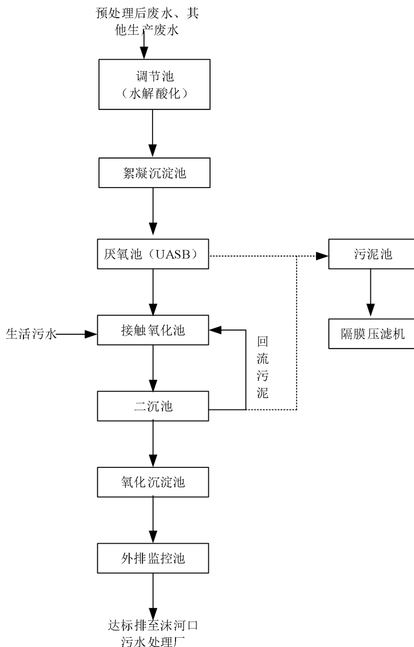
图 7.1.2-2 海华科技综合污水处理站处理工艺流程图
