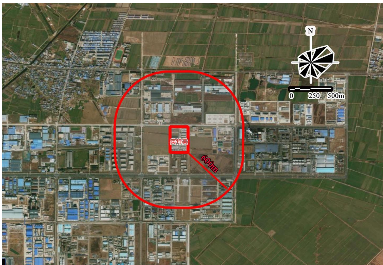
图 5-2-1.1 拟建项目环境防护距离图
