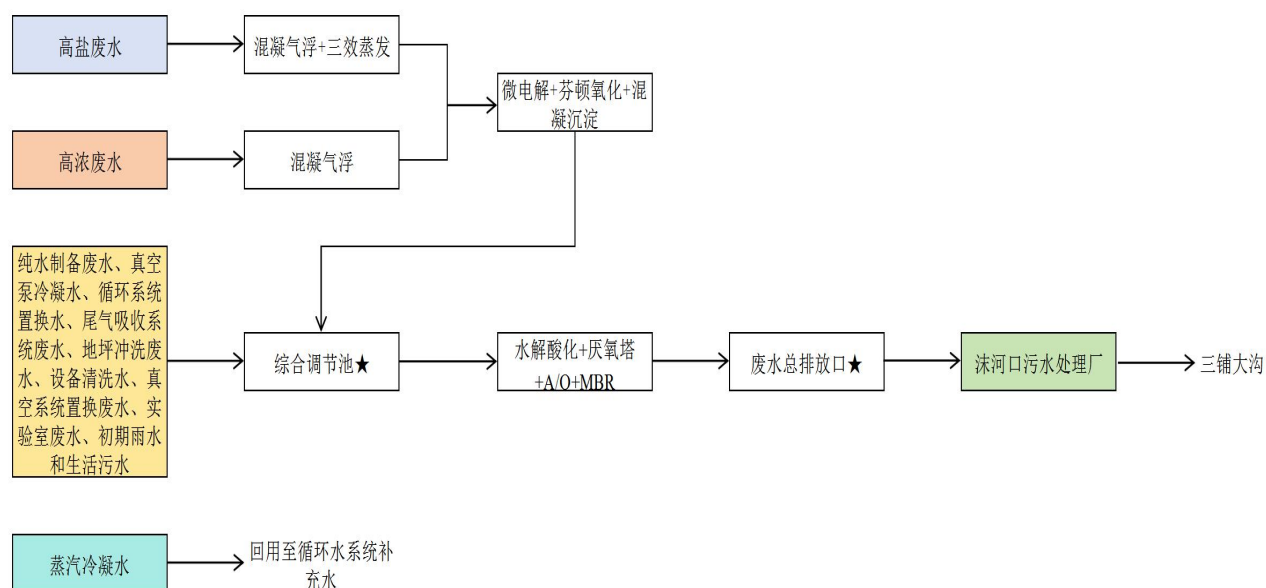
图 2-2-2.2 废水流向示意图及监测布点图（“★”表示为废水监测点位） 污水处理站处理工艺流程图见图 2-2-2.3。
