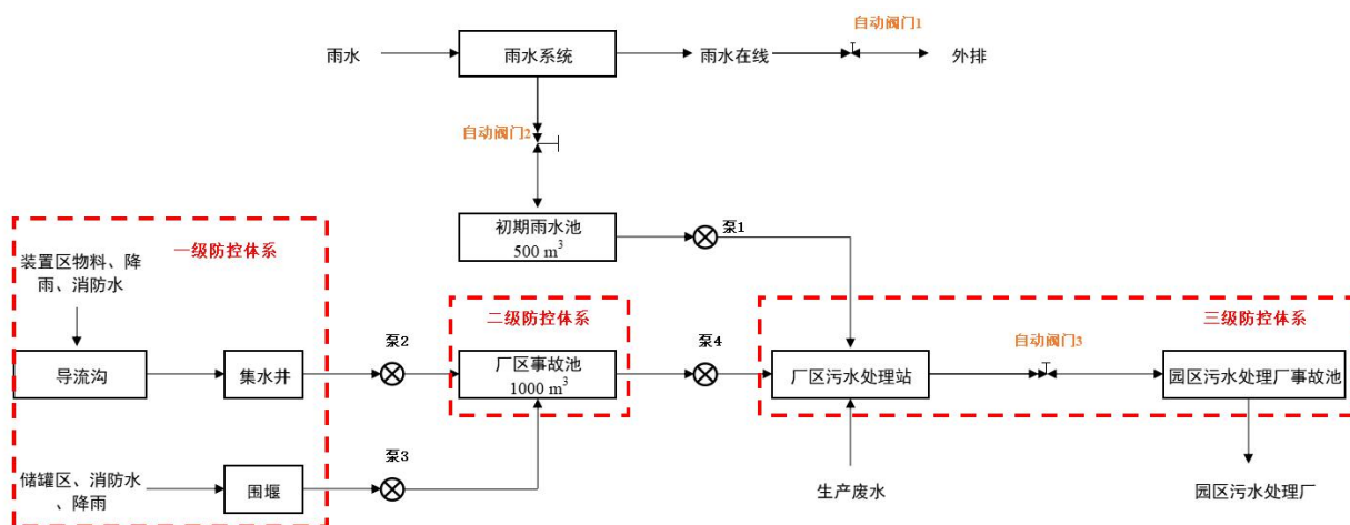
图 6-8-3.2 拟建项目事故状态下事故废水三级防控示意图
