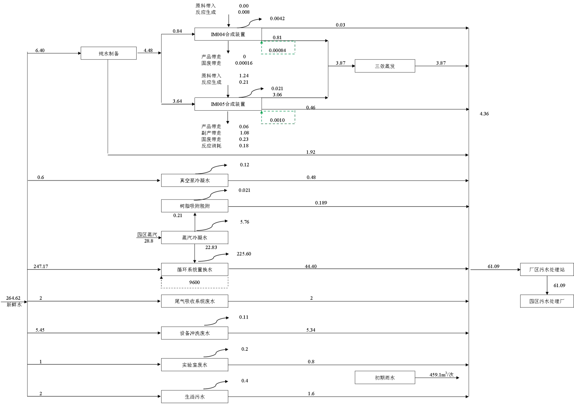
图 3-4-2.1 拟建项目水平衡图 (m³/d)
