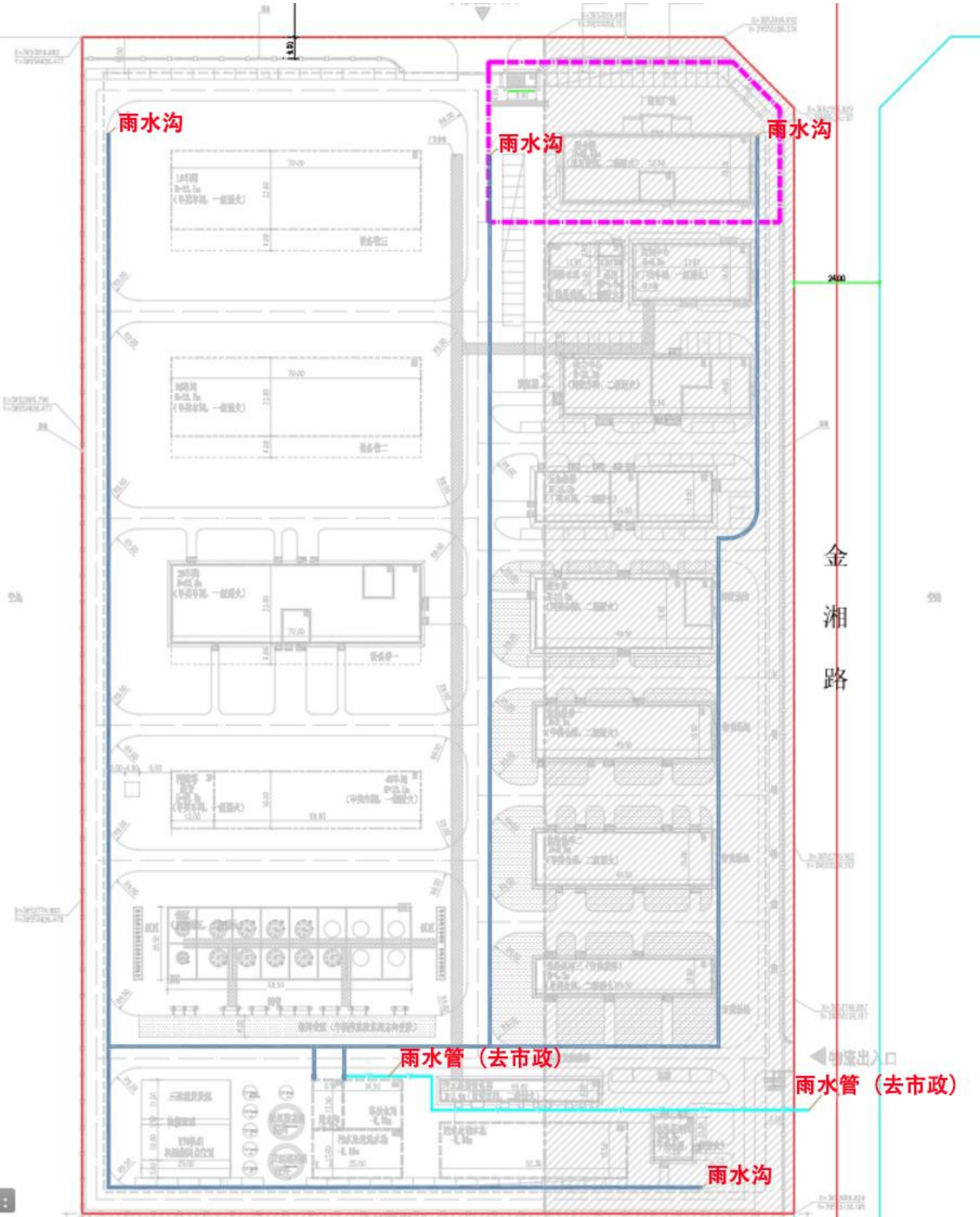
图 3-1-4.1 厂区雨水管线图
