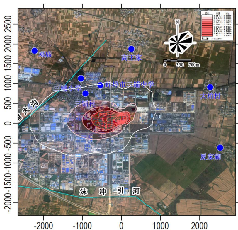
图 5-2-1.3 网格点处 PM 10 最大年均浓度贡献值等值线图 (μg/m 3 )
