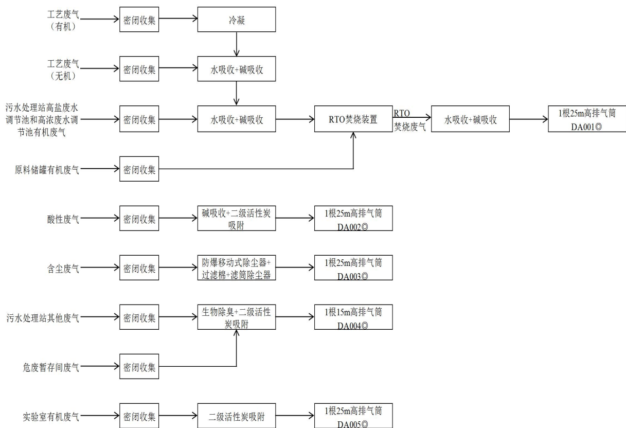
图 2-2-1.1 现有工程各类废气收集及处理措施示意图
