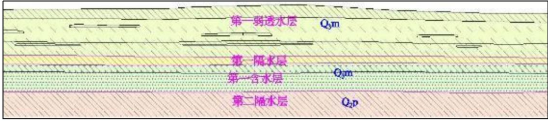
图 5-2-4.3 水文地质概化模型示意图
