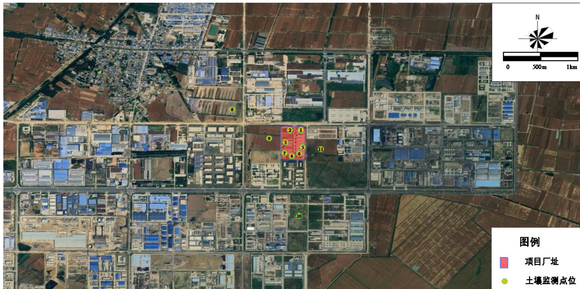
图 4-2-5.1 土壤环境质量现状监测布点示意图
