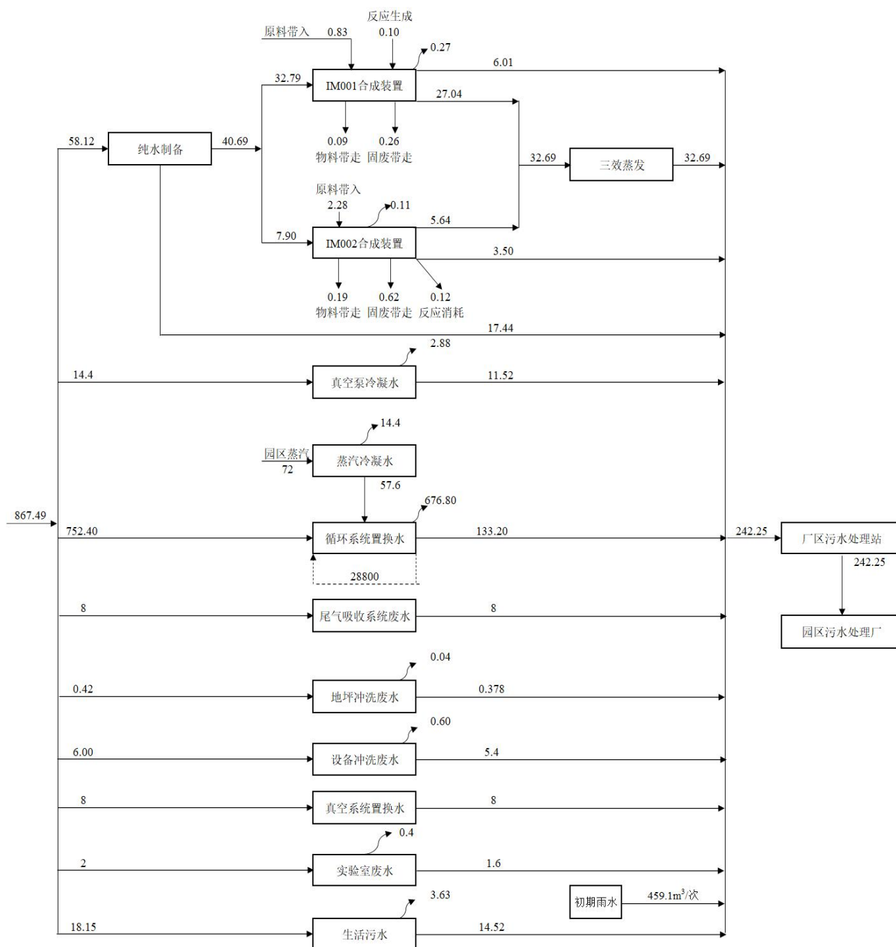
图 2-2-2.1 现有工程水平衡示意图 (单位: m 3 /d)
