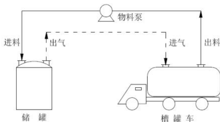
图 7.1.3-5 物料进入储罐时的排放控制措施
