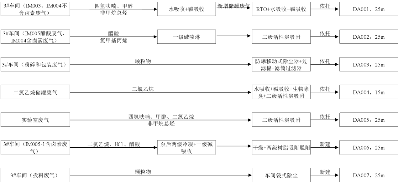
图 7.1.3-1 拟建项目各类废气收集及处理措施示意图
