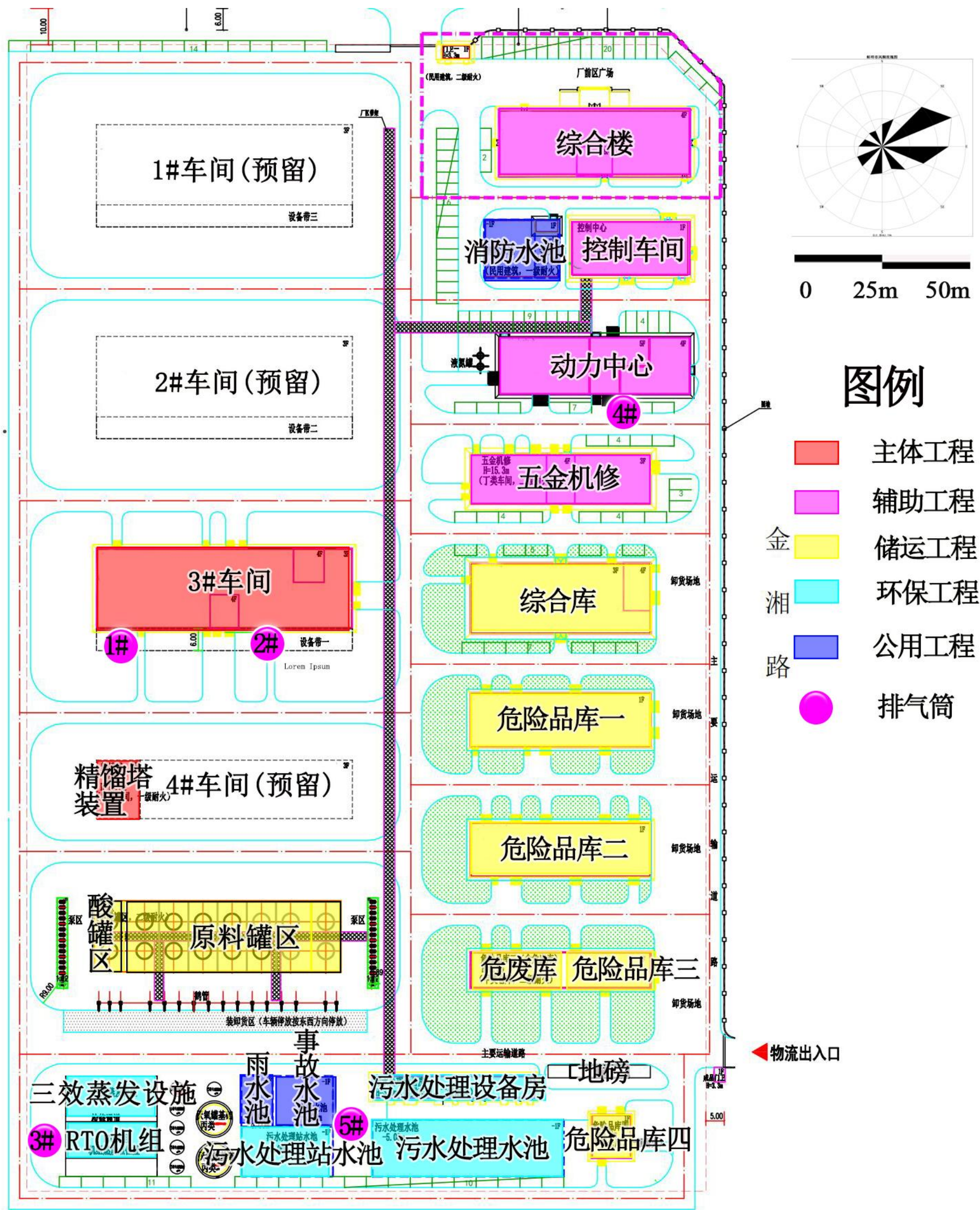
图 3-1-9.1 厂区总平面布置图
