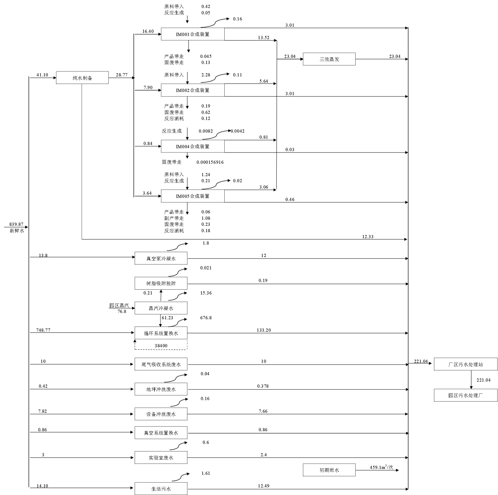
图 3-4-2.2 拟建项目建成后全厂水平衡图 (m³/d)
