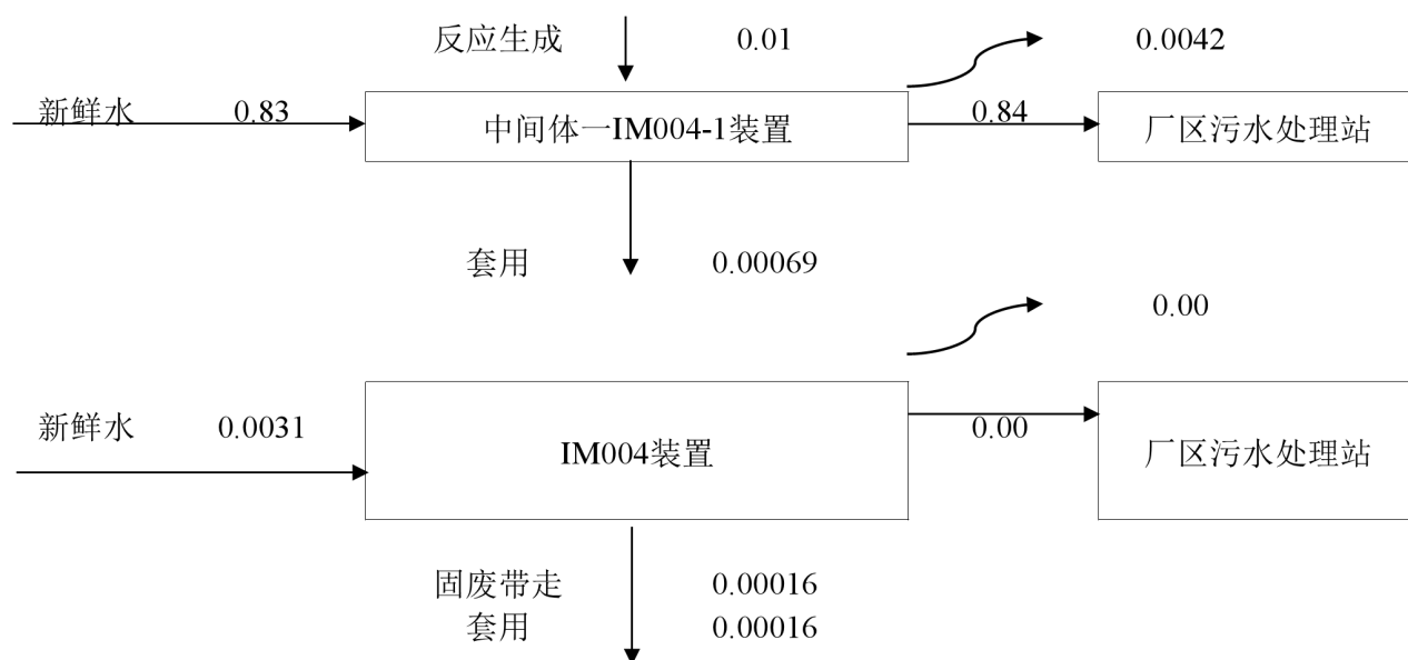
图 3-2-3.5 IM004 装置水平衡示意图 (m³/d)
