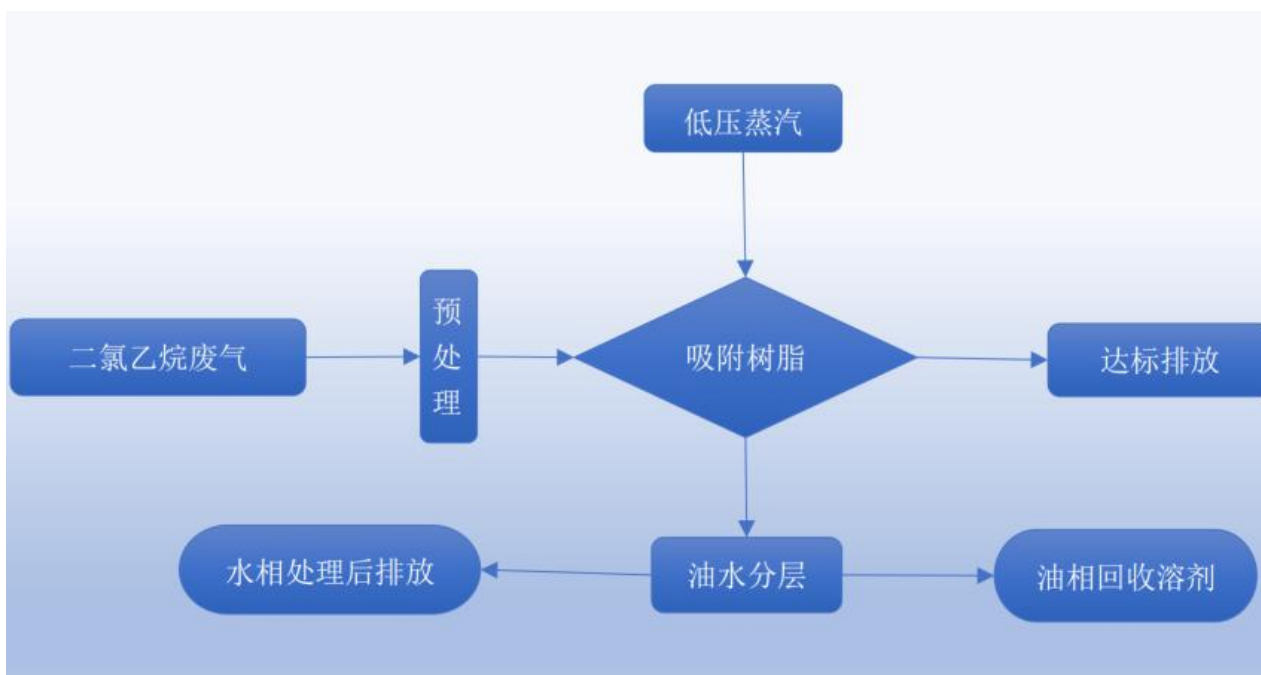
图 7.1.3-4 树脂吸附工艺流程方框图
