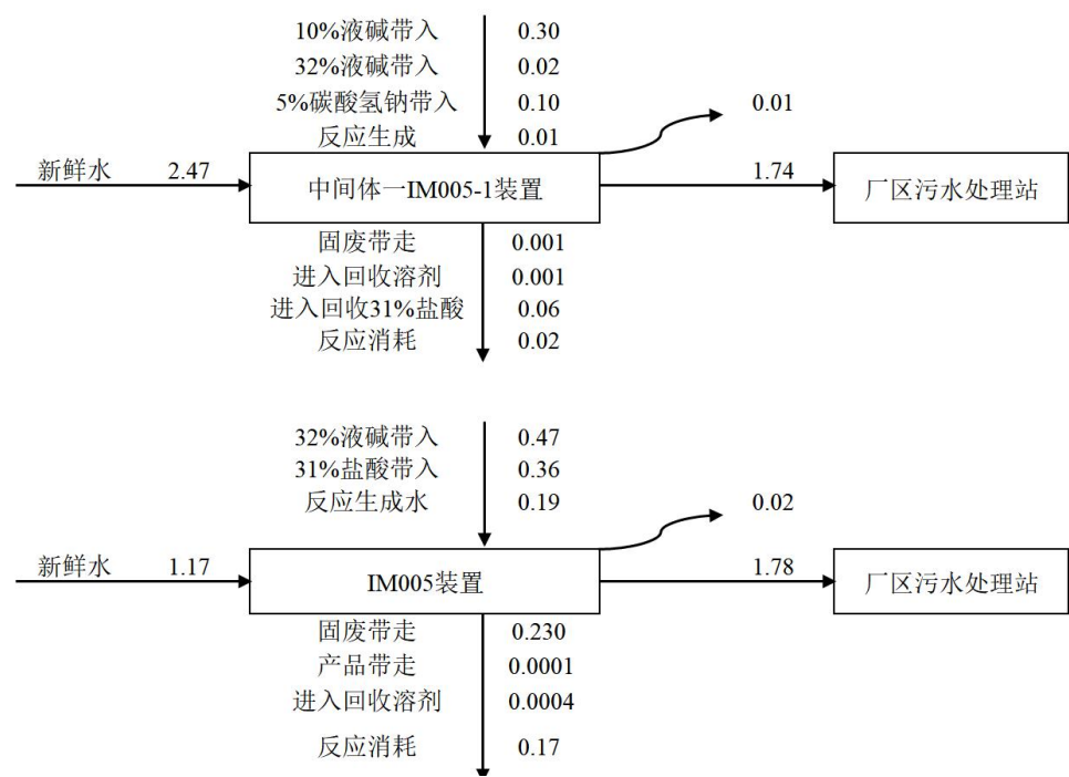
图 3-2-4.5 IM005 装置水平衡示意图 (m³/d)
