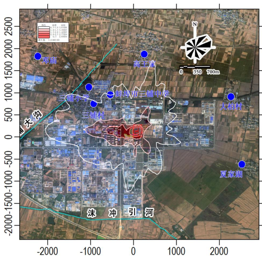
图 5-2-1.2 网格点处 PM 10 最大日均浓度贡献值等值线图 (μg/m 3 )
