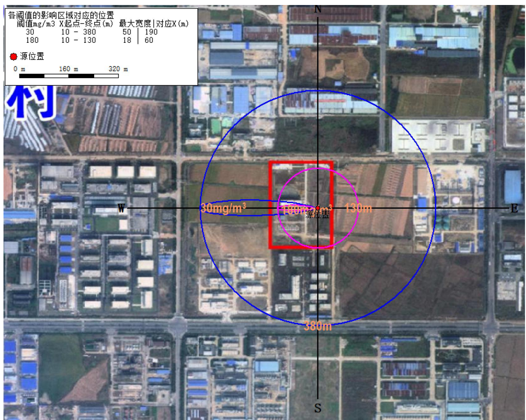
图 6-7-1.3 不同气象条件下乙酰氯预测浓度达到不同毒性终点浓度最大影响范围分布图
