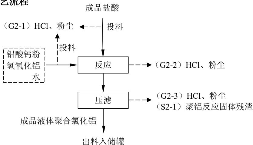
图 3.6-4 聚合氯化铝生产工艺流程图
