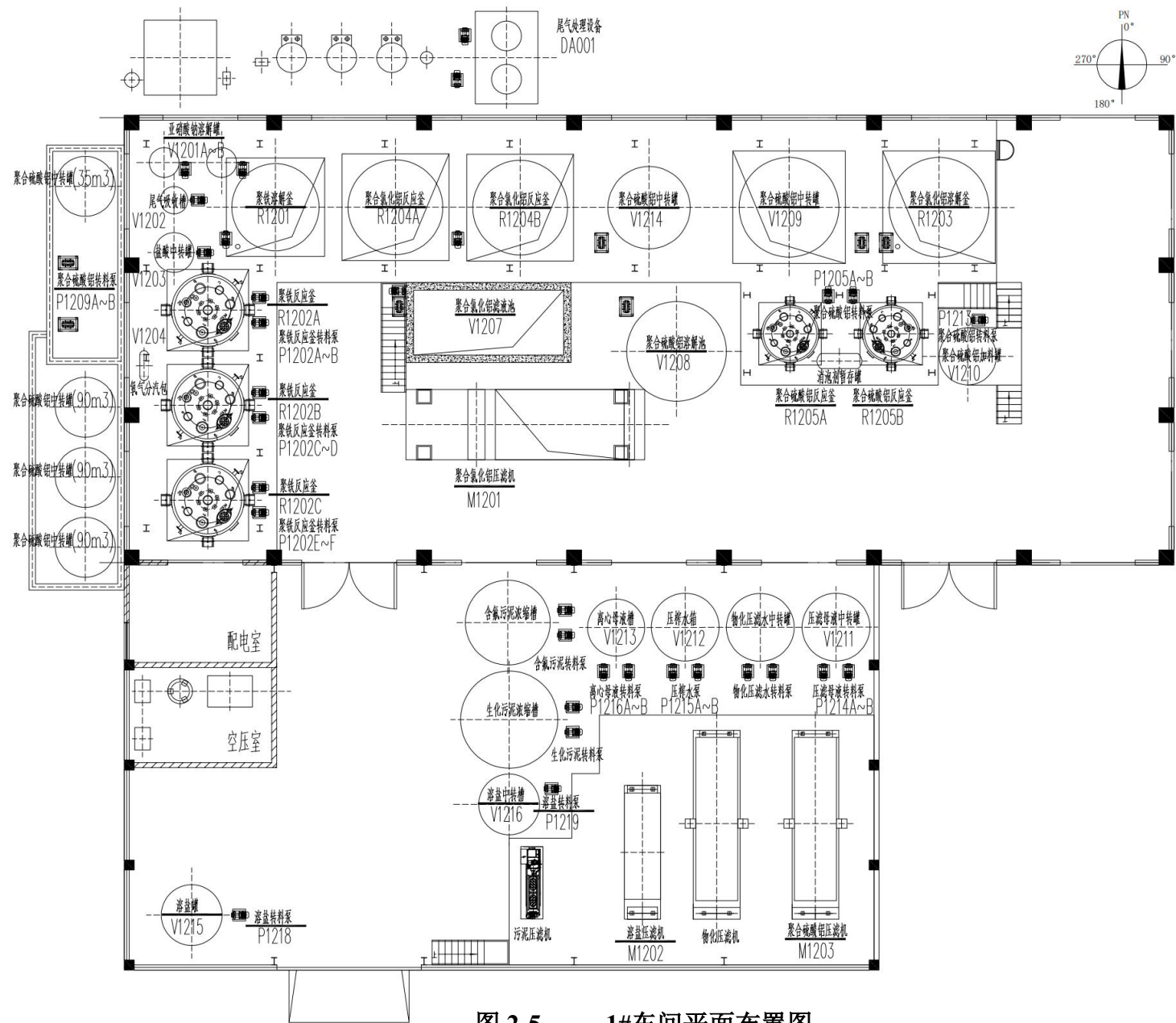
图 2-5 1#车间平面布置图
