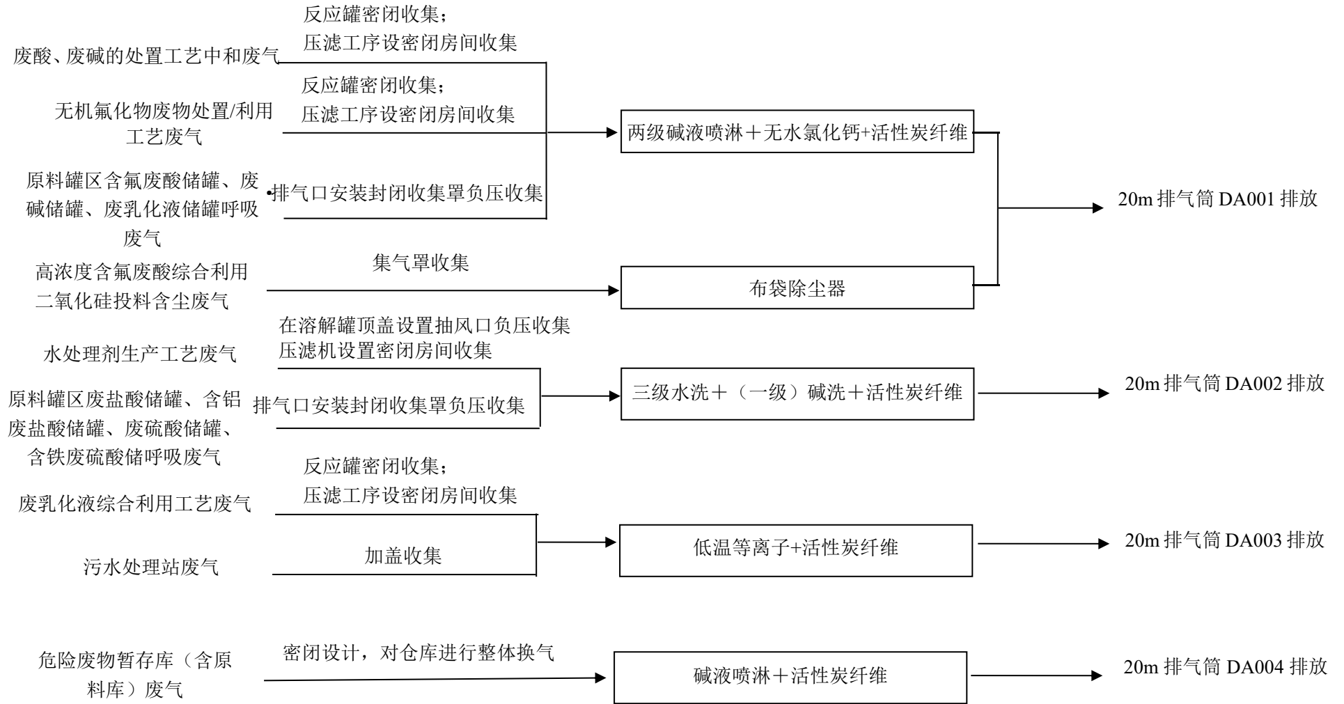
图 3.1-6 项目废气收集、处置示意图
