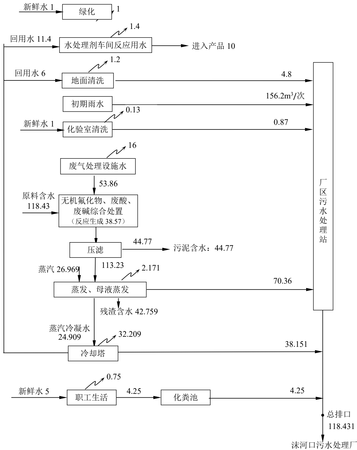
图 3.7-1 项目全厂给排水水量平衡图 (单位: t/d)
