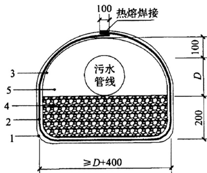
图 5-12 地下管道高密度聚乙烯（HDPE）膜防渗层示意图
