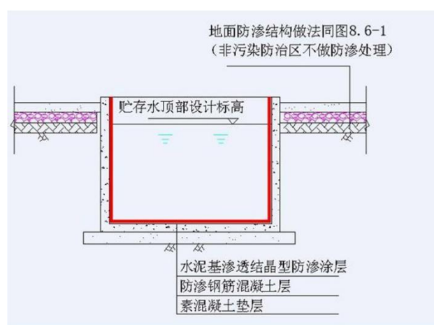
图 6-10 污水池防渗层结构图
