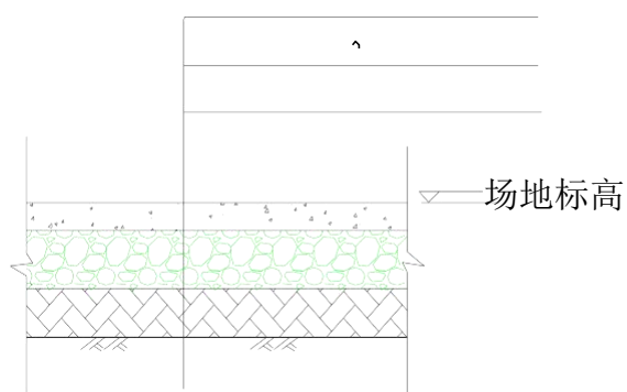
图 6-14 一般污染防治区典型防渗结构图
