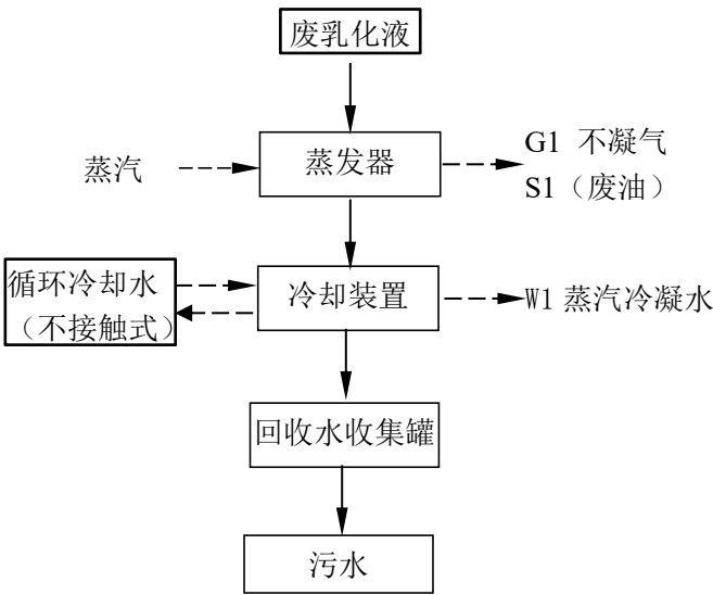
图 3.1-5 废乳化液综合利用工艺流程框图
