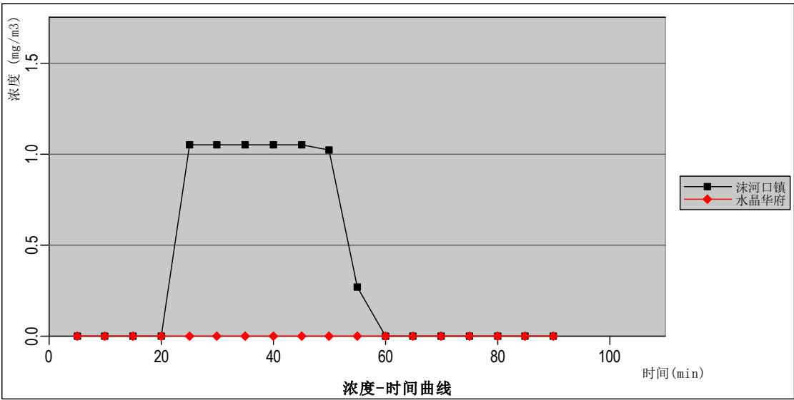
图 5-24 最常见气象条件下含氟废酸泄漏主要关心点浓度随时间变化情况图
