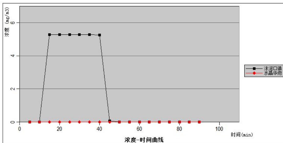
图 5-28 最常见象条件下主要关心点浓度随时间变化情况图
