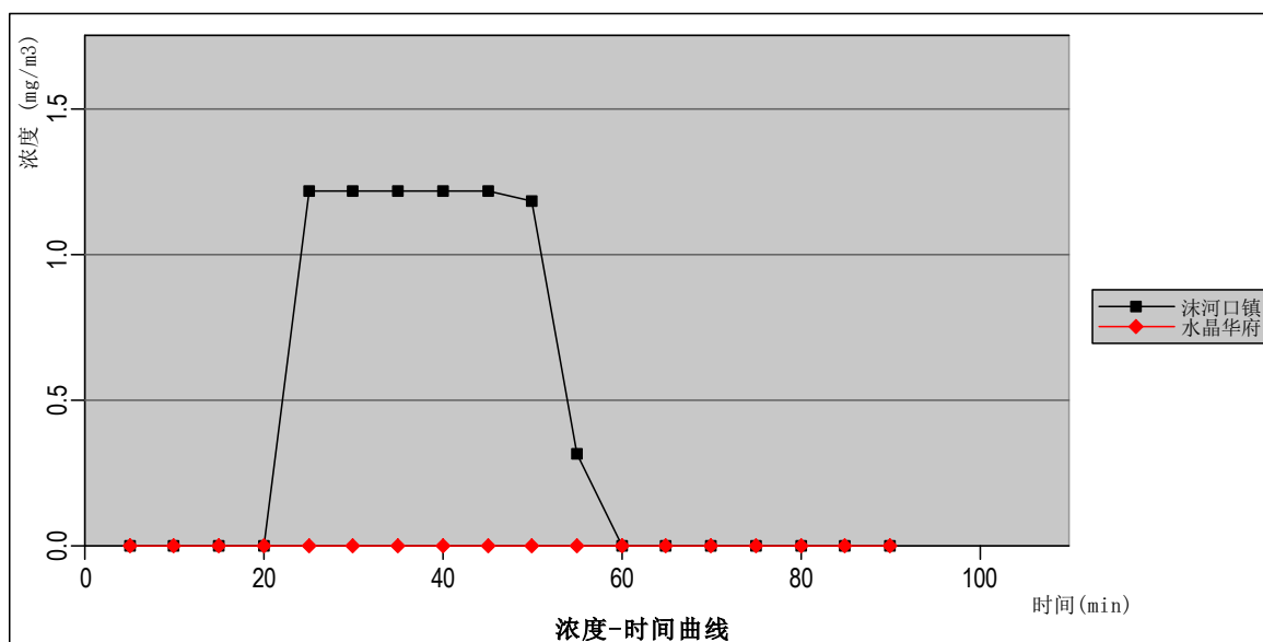
图 5-20 最常见气象条件下废盐酸泄漏主要关心点浓度随时间变化情况图
