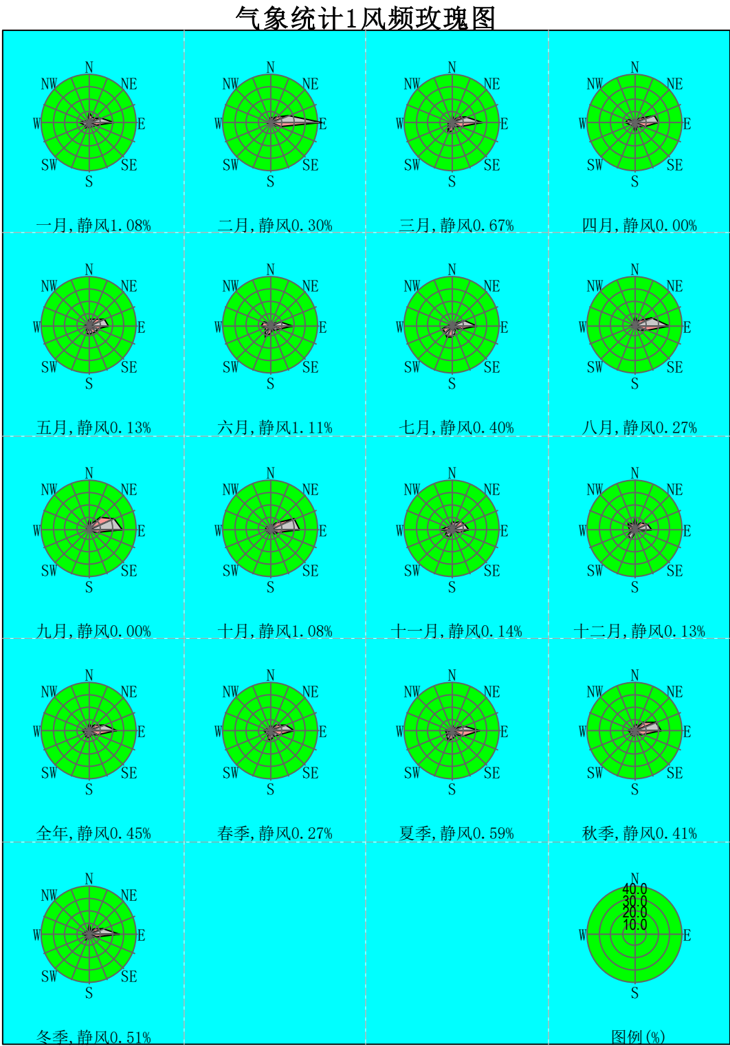
图5.2-12 2023 年蚌埠气象台站风向频率玫瑰图
