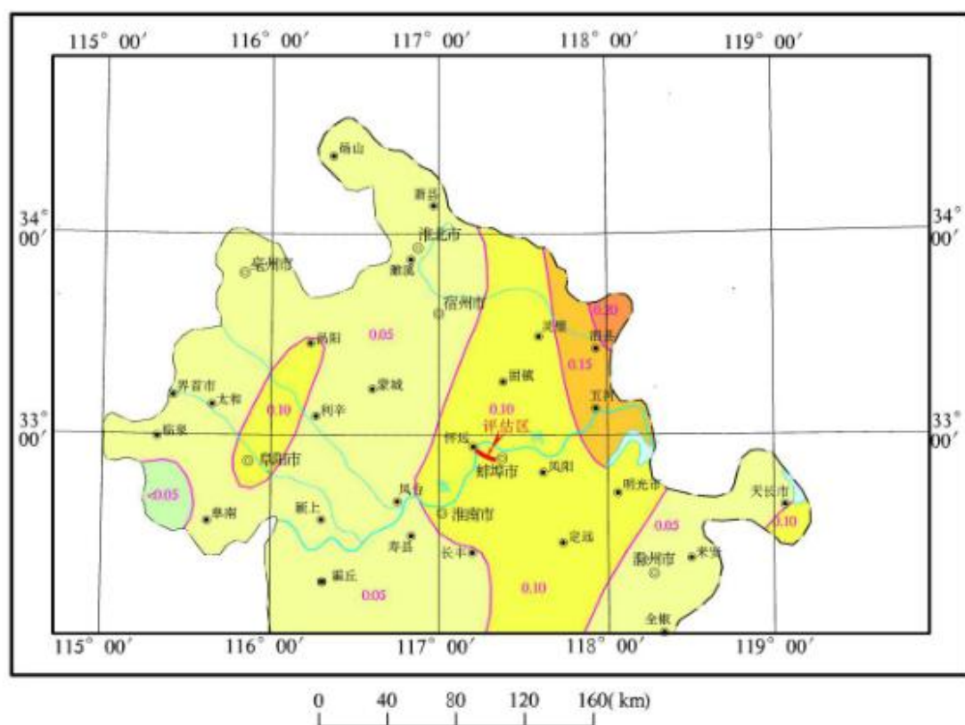
图 5-6 地震动峰值加速度区划图
