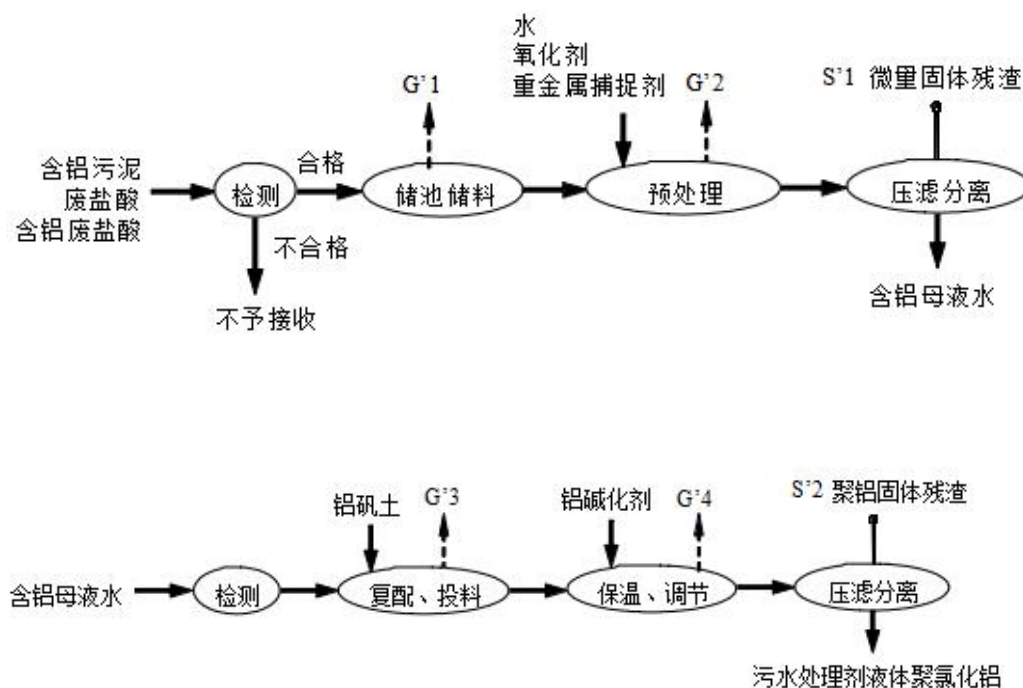
图 6-4 永葆公司聚氯化铝生产工艺图
