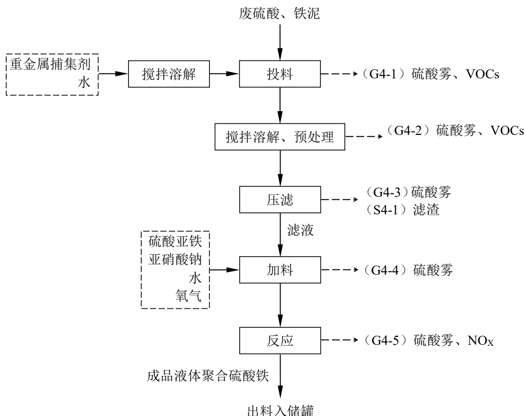
图 3.6-6 废硫酸、含铁污泥综合利用处置工艺流程图
