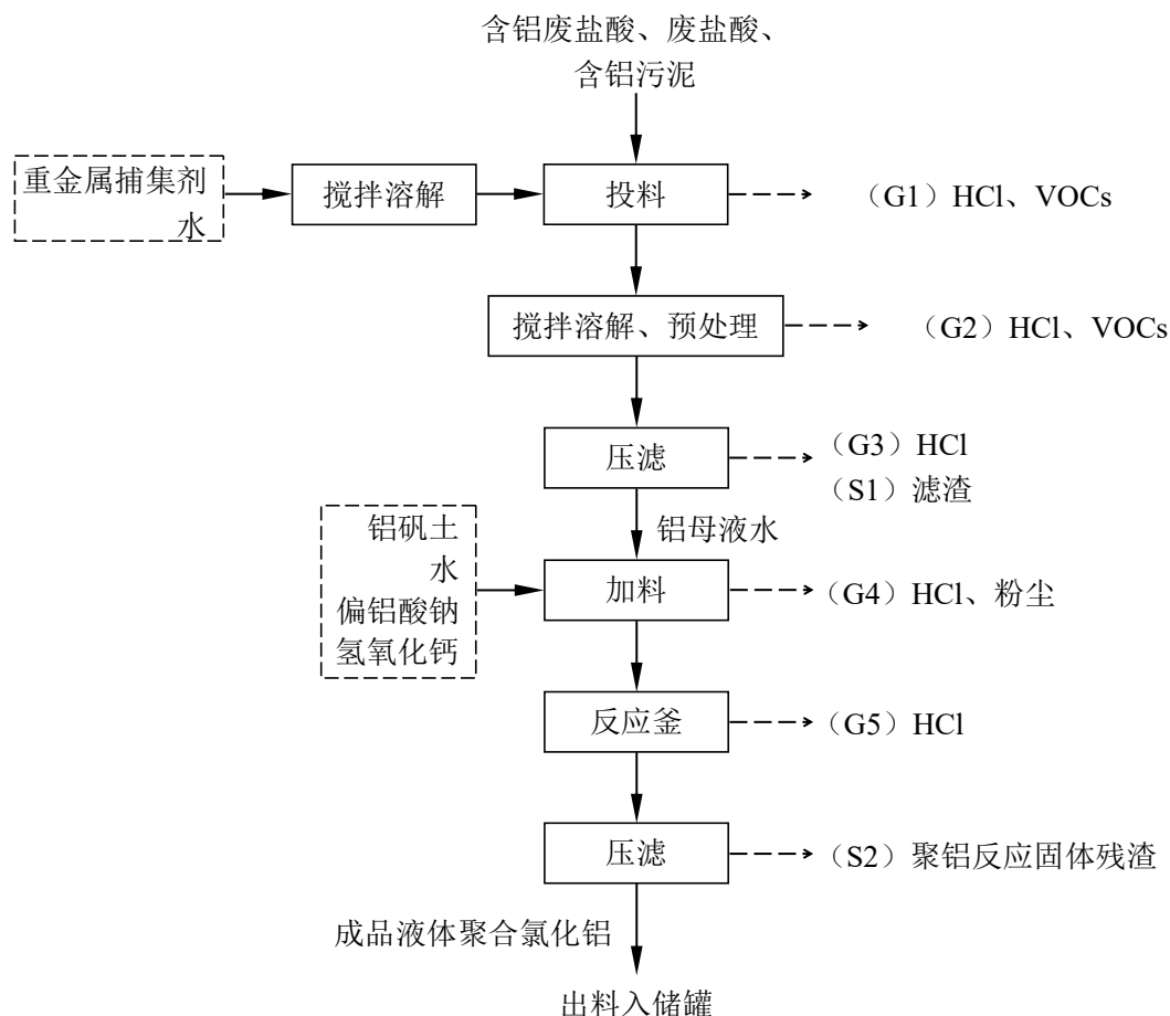
图 3.1-2 含铝废盐酸、废盐酸、含铝污泥综合利用处置工艺流程图
