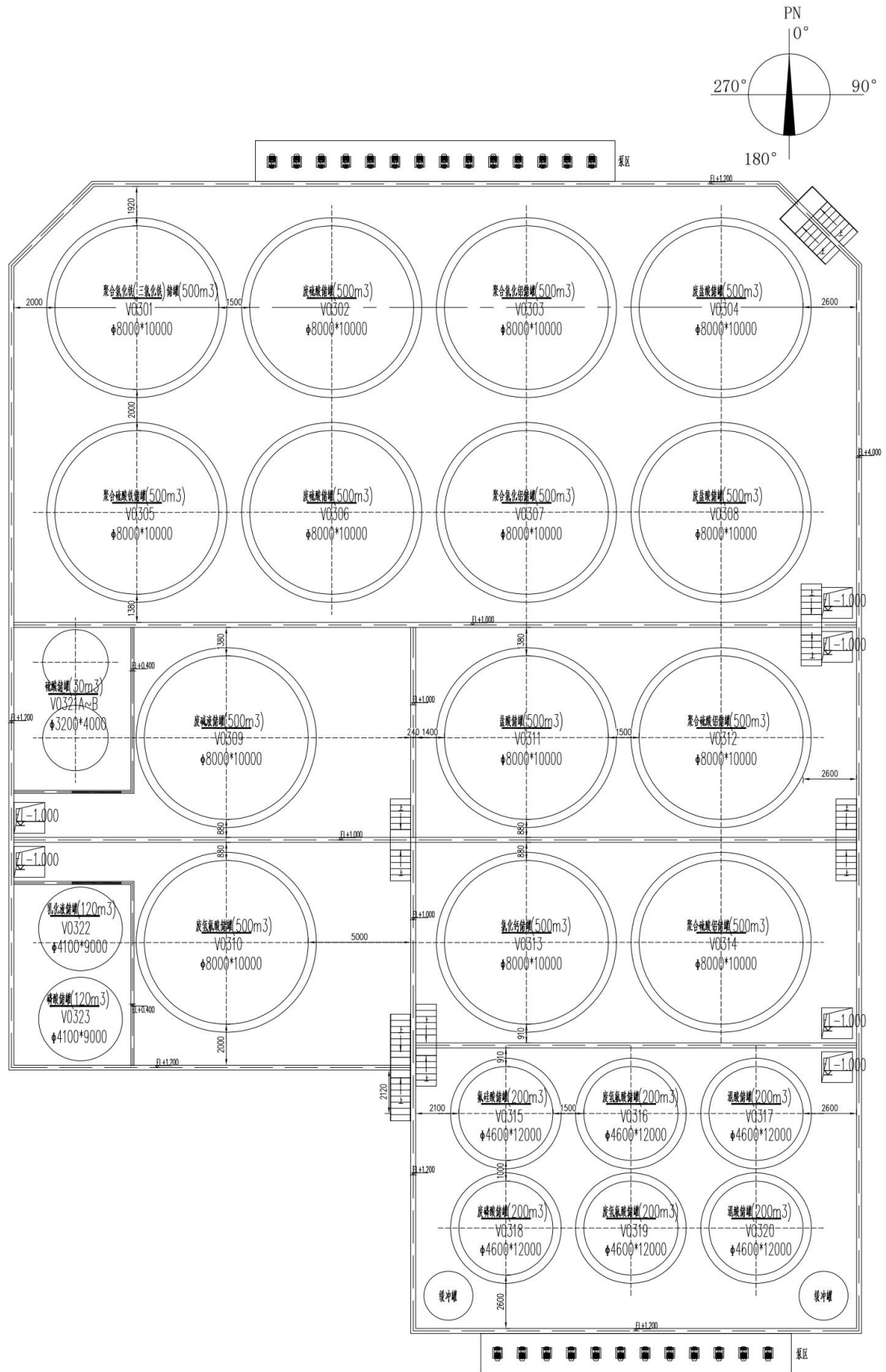
图 2-7 罐区平面布置图
