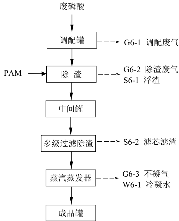
图 3.6-8 废磷酸提纯工艺流程框图
