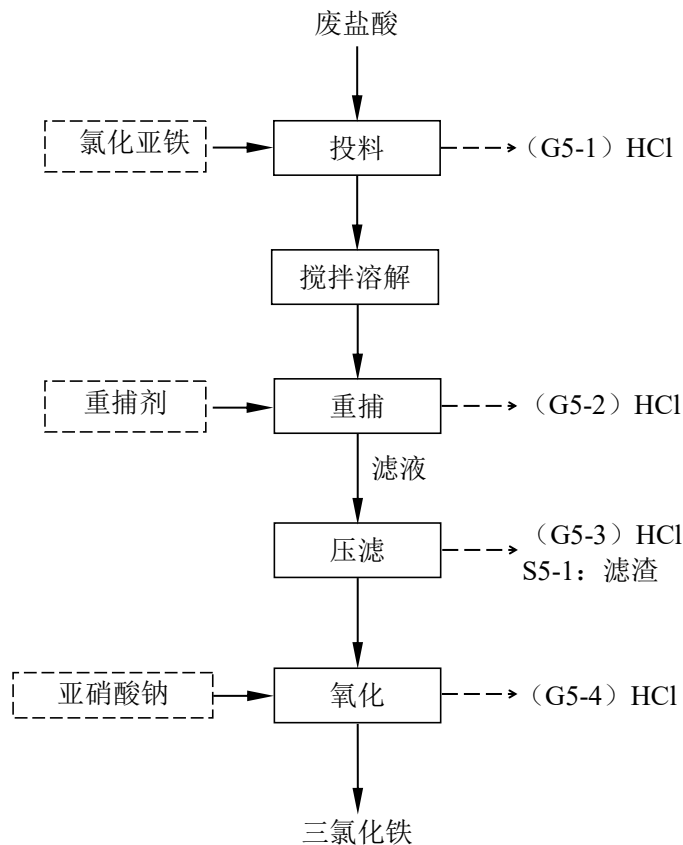
图 3.6-7 废盐酸综合利用处置工艺流程图
