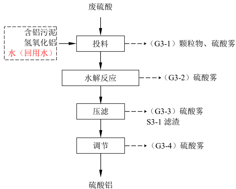
图 3.6-5 含铝污泥、废硫酸综合利用处置工艺流程图
