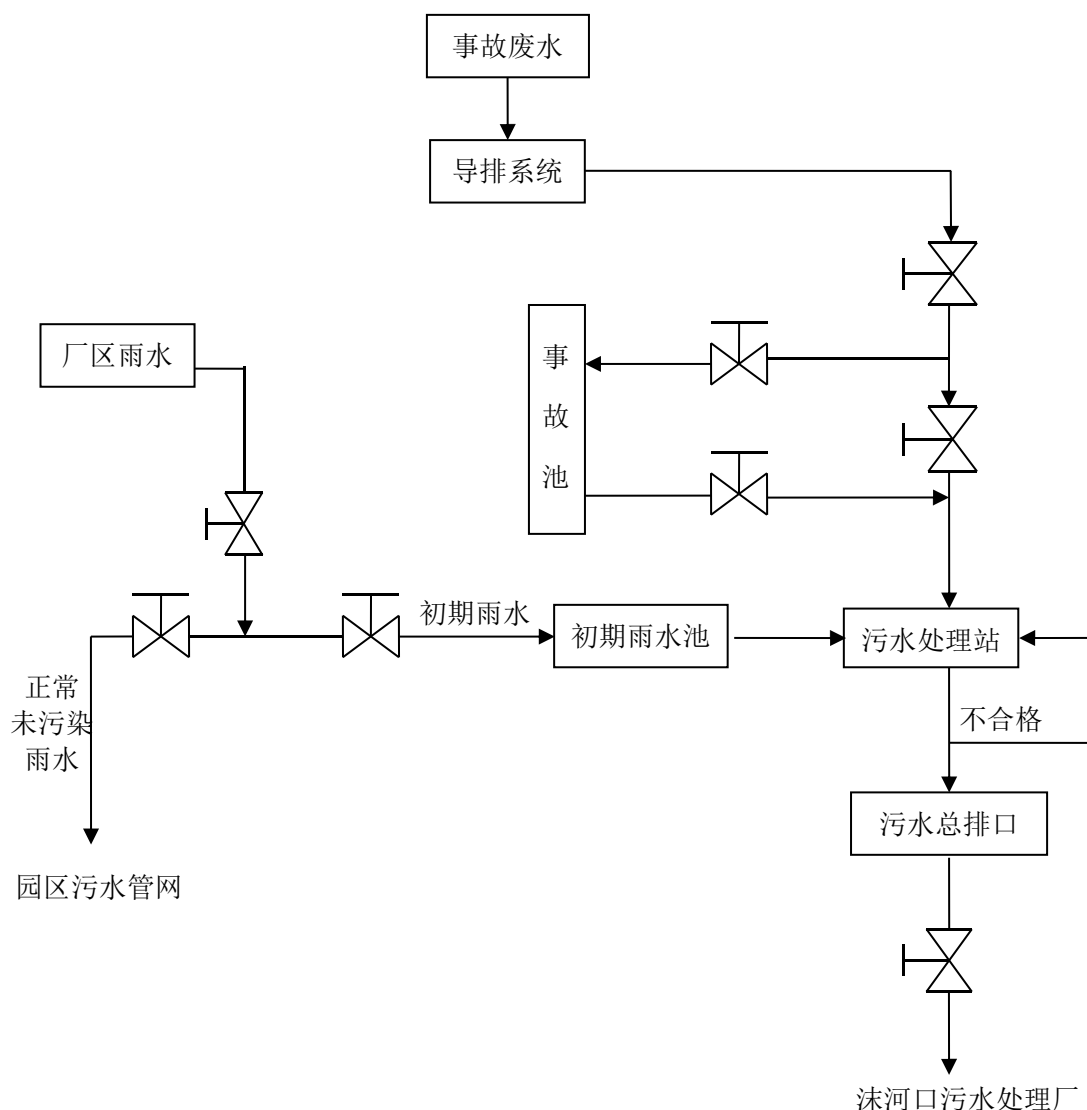
图 5-29 事故废水切断措施示意图
