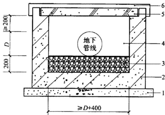
图 5-13 抗渗钢筋混凝土管沟防渗层示意图
