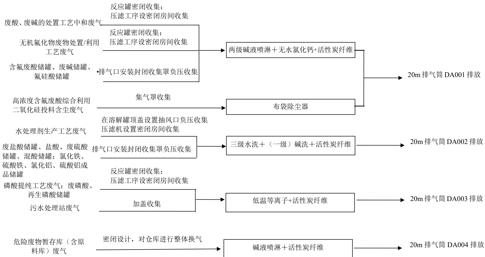
图 6-1 项目废气收集、处置示意图
