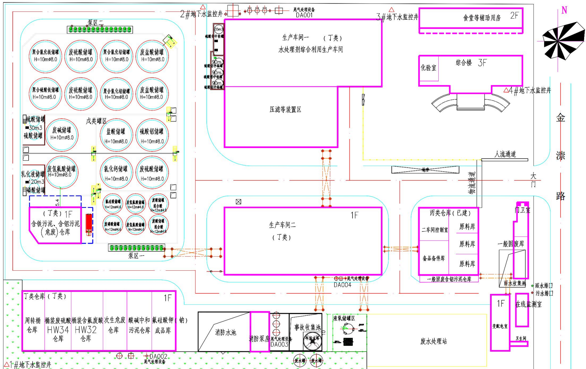
图 2-4 厂区平面布置图
