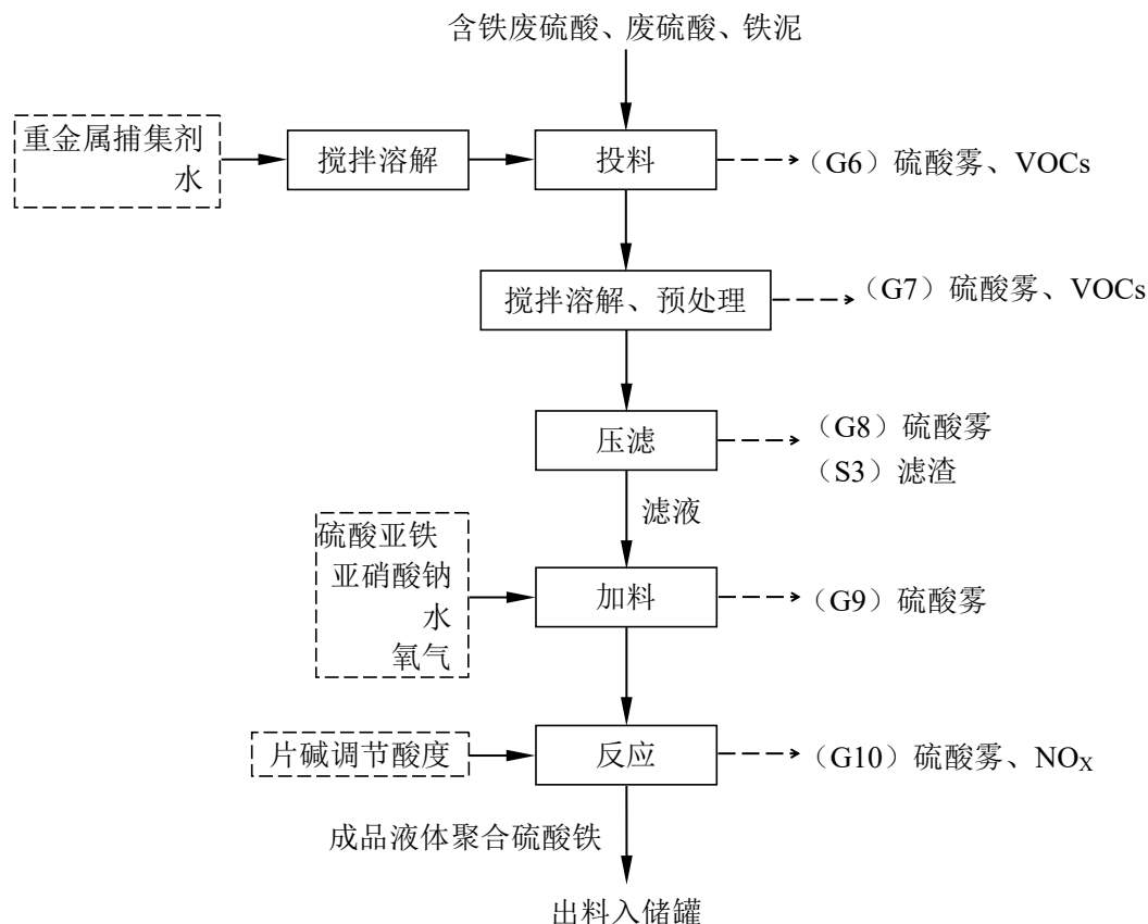
图 3.1-3 含铁废硫酸、铁泥利用处置工艺流程图
