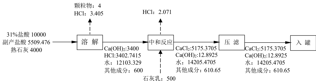
图 3.6-11 氯化钙物料平衡图
