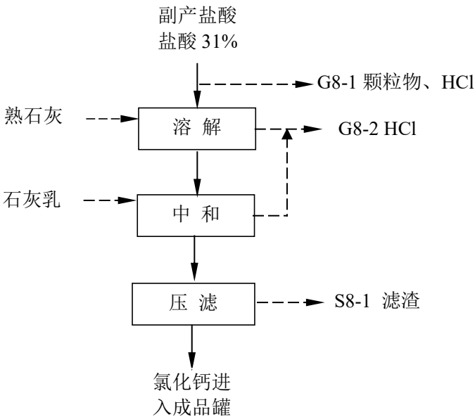
图 3.6-10 副产盐酸综合利用生产工艺流程及产排污节点
