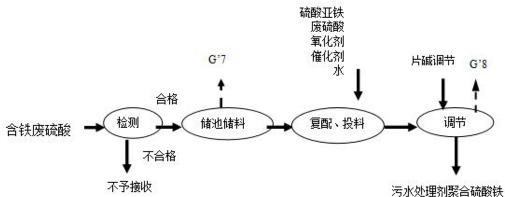
图 6-5 永葆公司聚合硫酸铁生产工艺图
