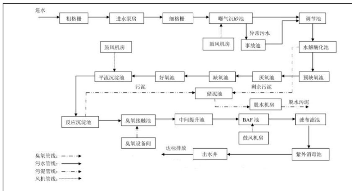
图 6-7 沫河口工业园污水处理厂工艺流程图
