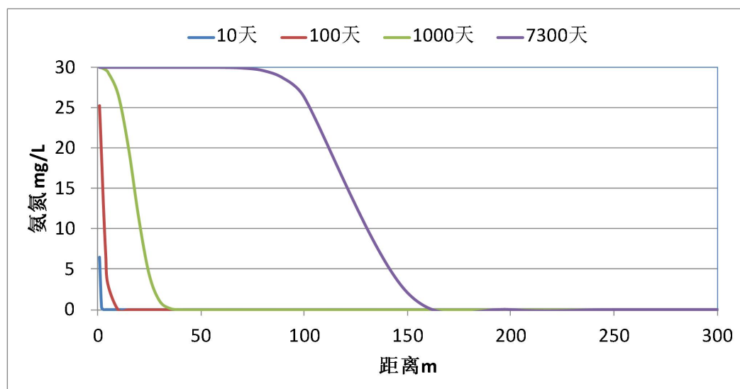
图 5-10 非正常工况下氨氮浓度变化结果图
