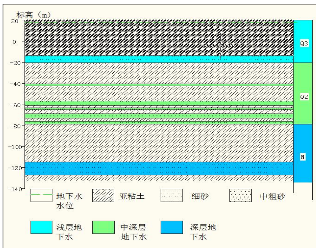
图4.1-2 工作区水文地质剖面图
