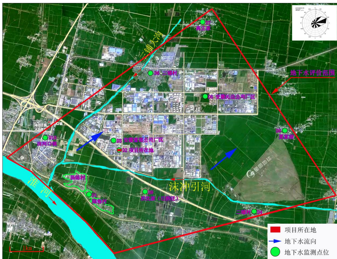
图 5-8 地下水评价范围图
