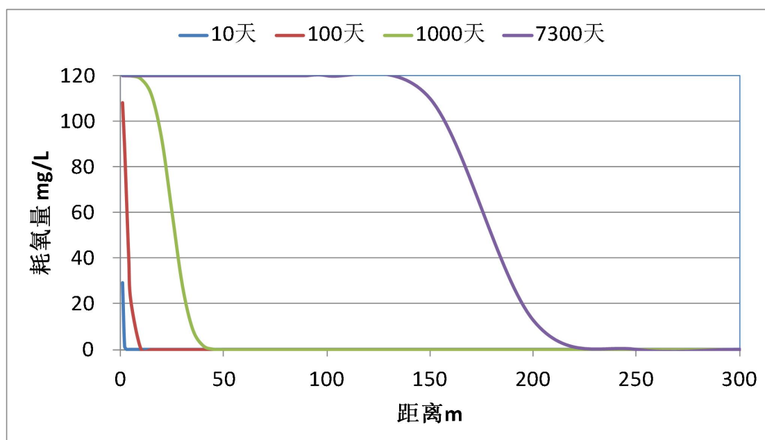
图 5-9 非正常工况下耗氧量浓度变化结果图
