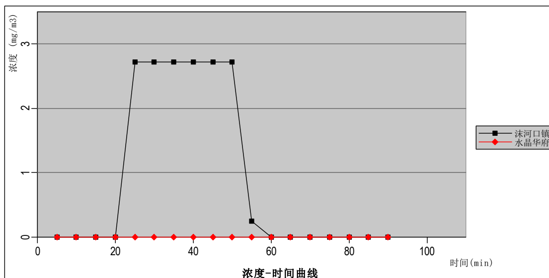
图 5-22 最不利气象条件下含氟废酸泄漏主要关心点浓度随时间变化情况图
