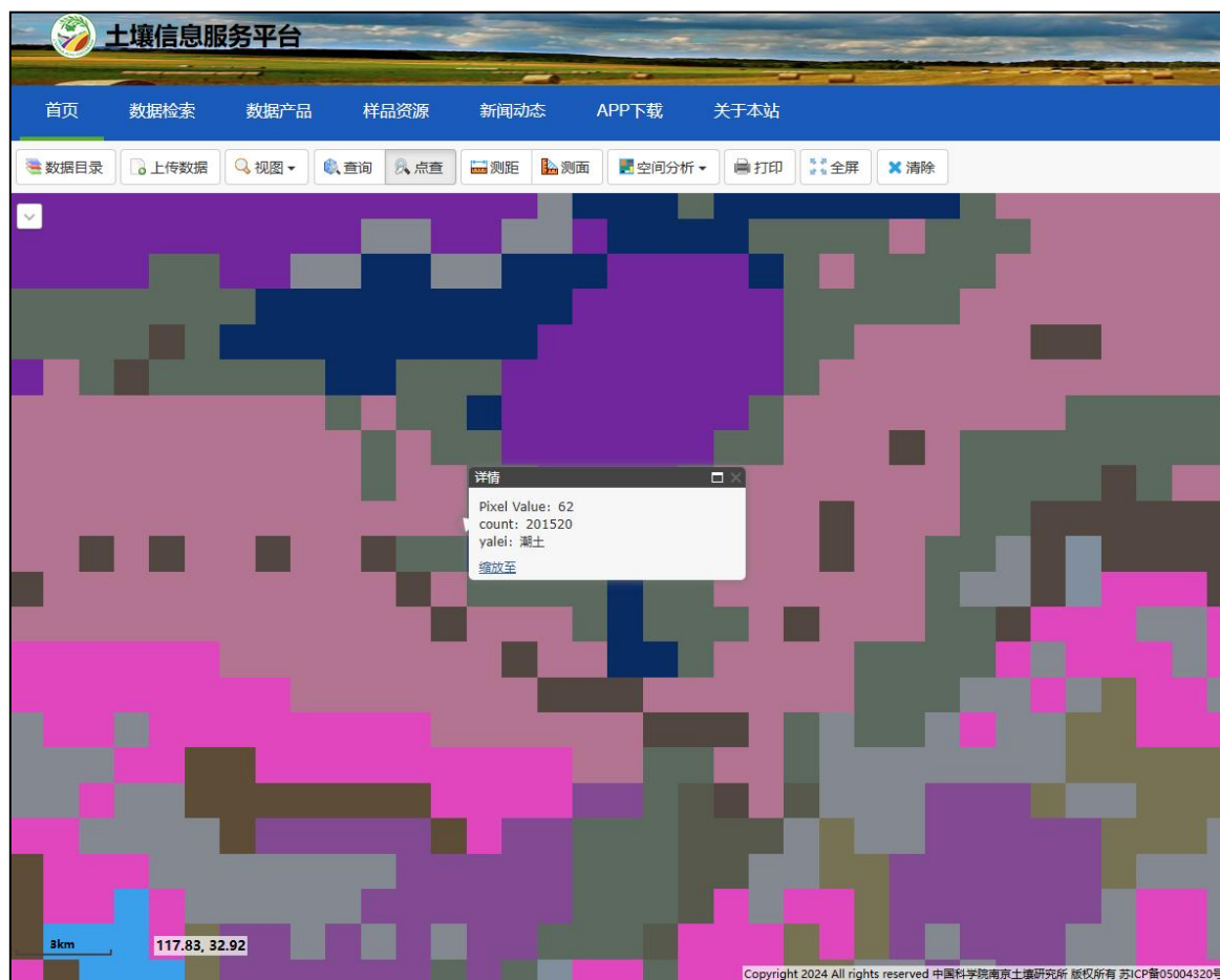
图 5-31 土壤调查范围土壤类型图
