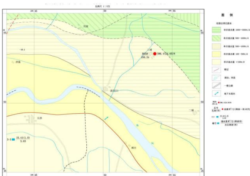
图 5-7 区域环境水文地质图(1/5 万)
