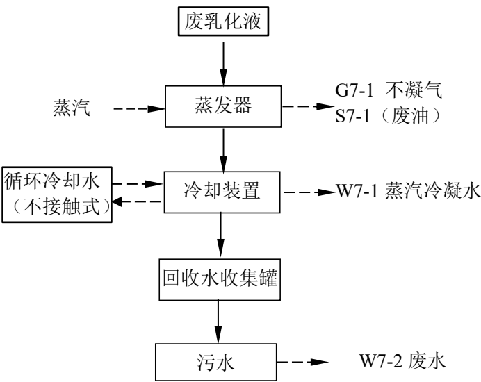
图 3.6-9 废乳化液综合利用工艺流程框图
