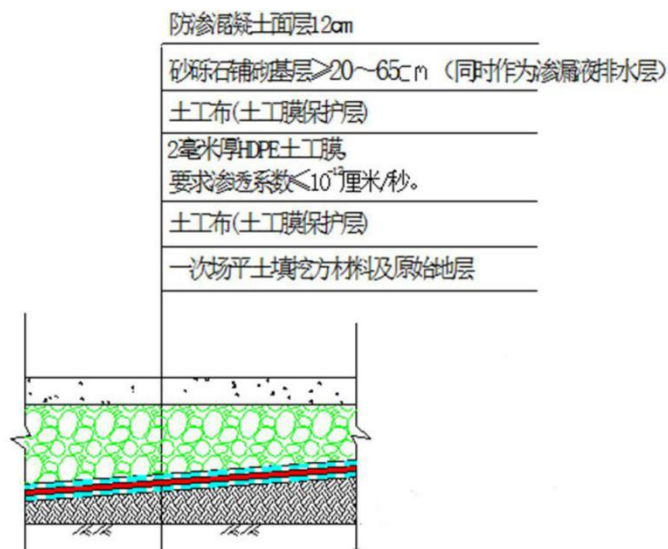
图6-9 生产车间防渗层设计方案
