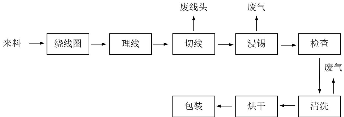
图 2 本项目工艺流程图
